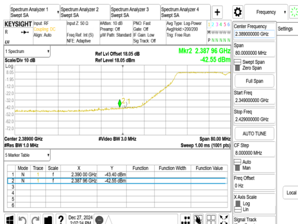
802.11n_40MHz_Chain1_2432MHz
