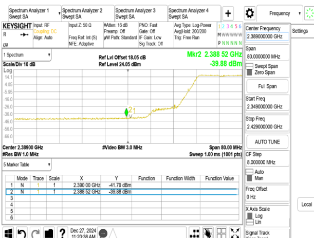
802.11n_20MHz_Chain0_2422MHz
