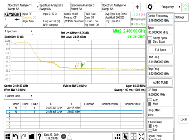
802.11n_20MHz_Chain1_2452MHz
