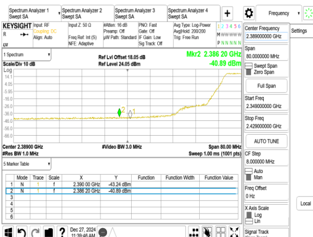
802.11n_20MHz_Chain1_2432MHz
