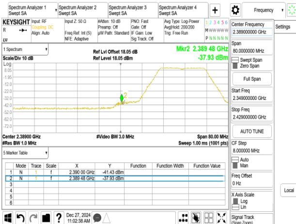
802.11n_20MHz_Chain0_2417MHz
