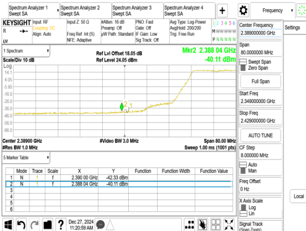
802.11n_20MHz_Chain1_2427MHz
