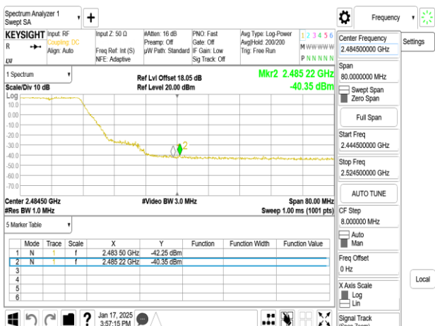
802.11g_20MHz_Chain0_2457MHz
