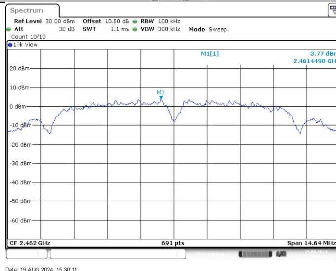
11B_Ant1_2462
