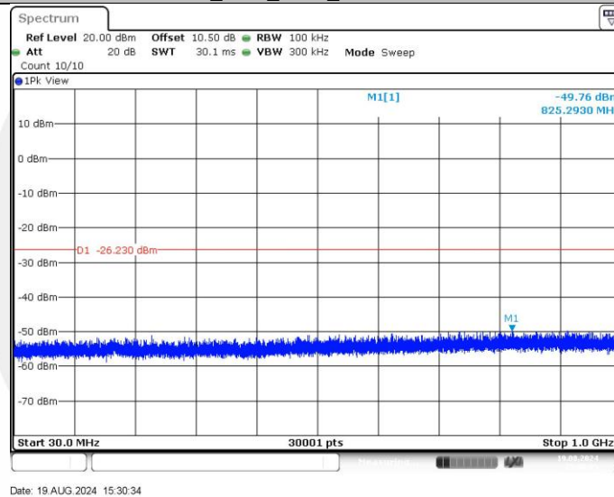
11B_Ant1_2462_30~1000
