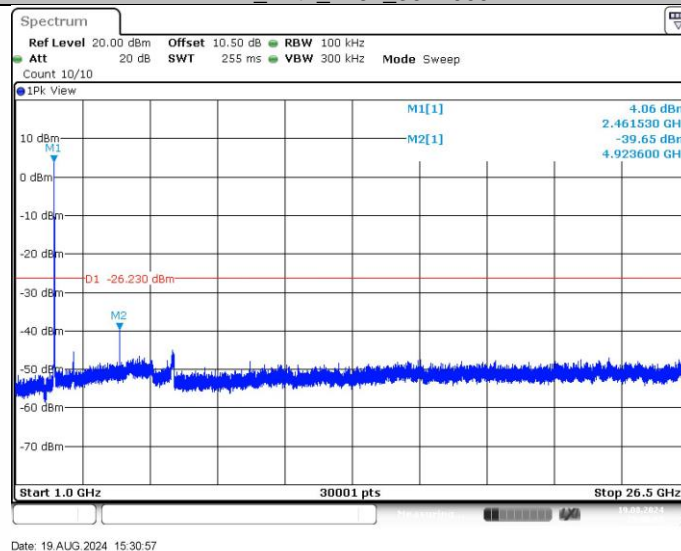
11B_Ant1_2462_1000~26500
