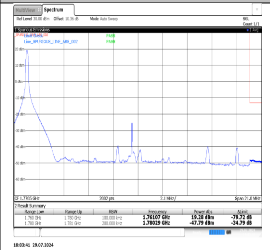
Band66-20MHz-QPSK-132572-1RB#0-PASS
