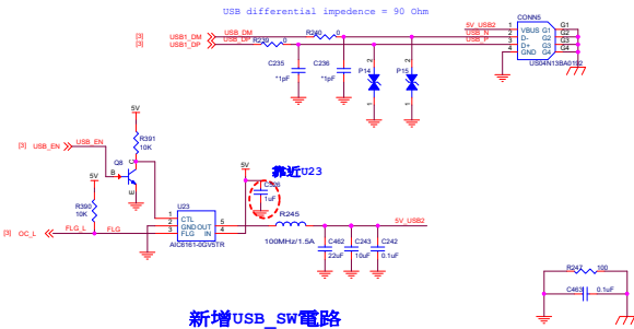
新增USB_SW電路
