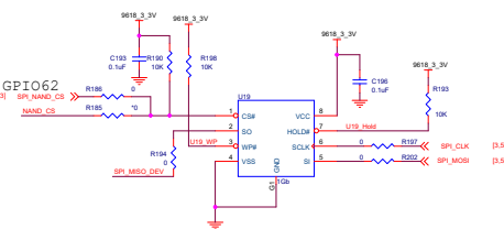
SPI NAND Flash_1Gbits
