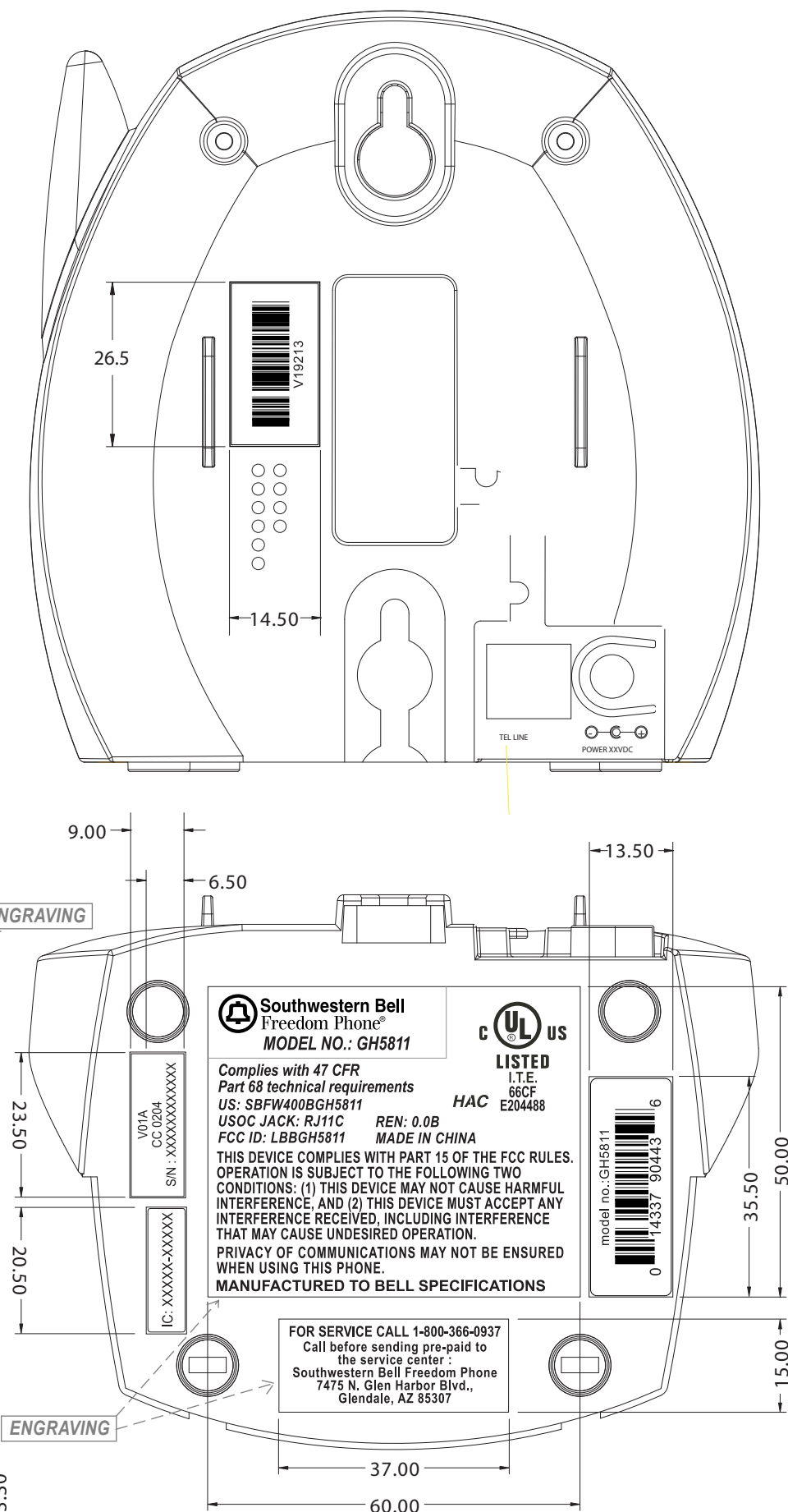
GH5811 BASE
