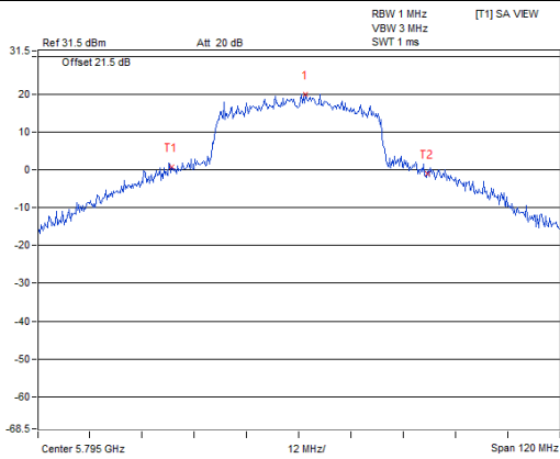
802.11ax (HE40)_Chain 1 / CH159
