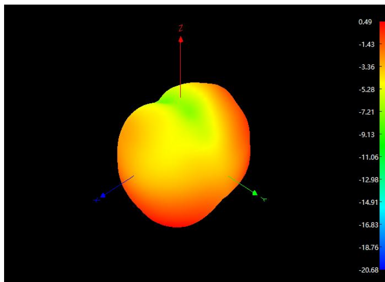
2500MHz 3D
