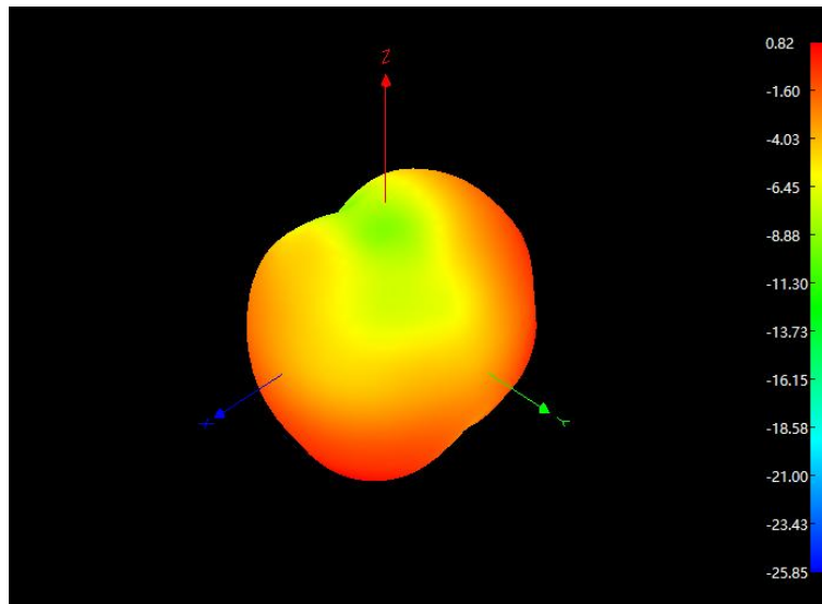
2450MHz 3D
