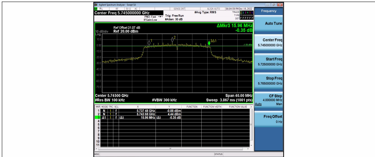
11N20MIMO Ant2 5745
