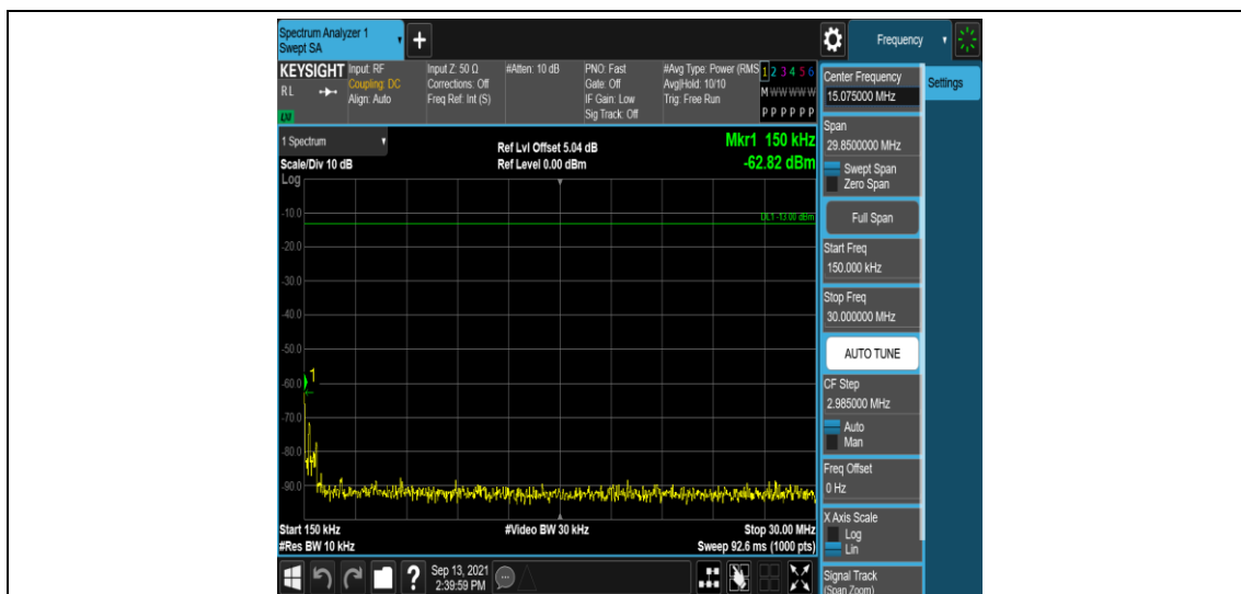
Band26-5MHz-QPSK-26915-1RB#0-Range2:0.15~30MHz
