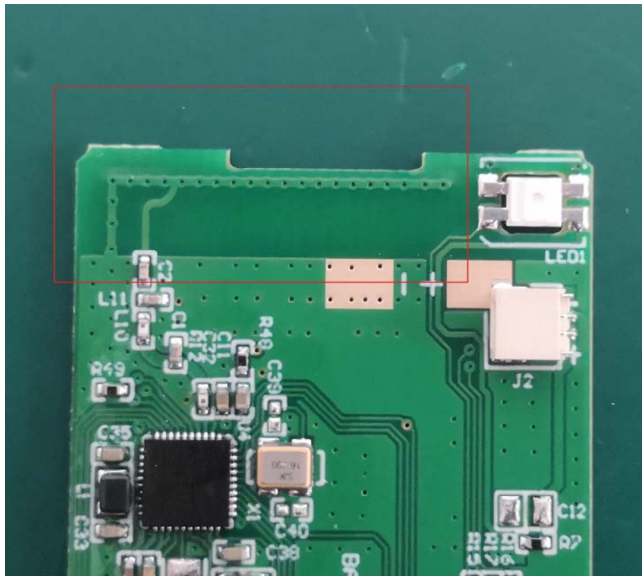
Antenna
