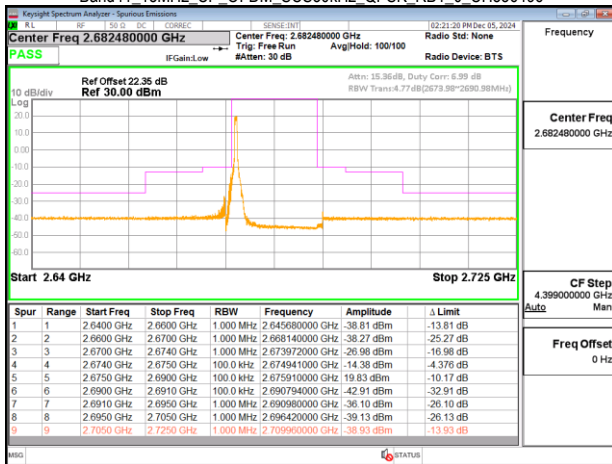
Band41_15MHz_CP_OFDM_SCS30kHz_QPSK_RB1_37_CH536496
