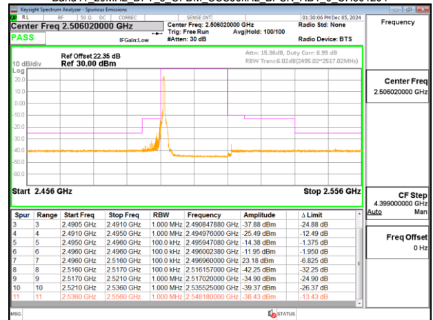
Band41_20MHz_DFT_s_OFDM_SCS30kHz_BPSK_RB1_50_CH501204
