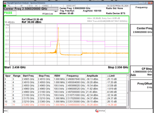
Band41 20MHz CP_OFDM_SCS30kHz QPSK RB1_50_CH501204
