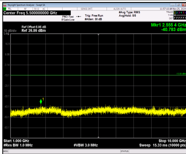
Band5-10MHz-QPSK-20525-1RB#0-Range2:1000~1 0000MHz
