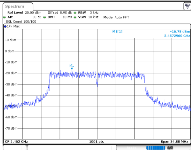
11N20SISO_Ant1_2462
