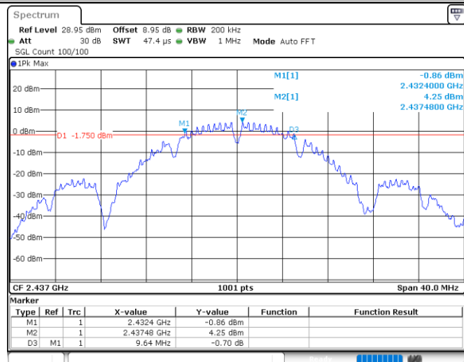
11B_Ant1_2437
