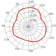
2500.000MHz E2
