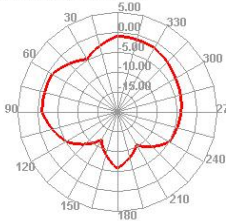
2400.000MHz E1
