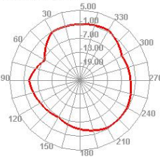
2400.000MHz E2
