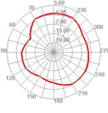
2450.000MHz E2
