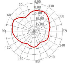
2500.000MHz E1
