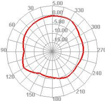
2450.000MHz E2
