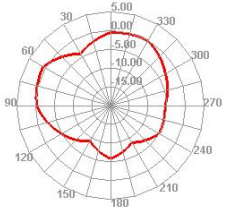
2450.000MHz E1
