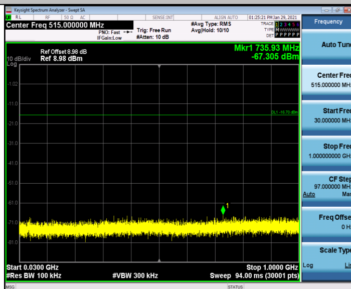
BLE_BT4.2_Ant1_2402_30~1000
