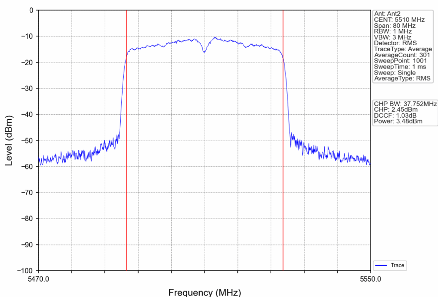
802.11ax(HEW40)_LCH_5510MHz_RU484_Left_Ant2_NTNV
