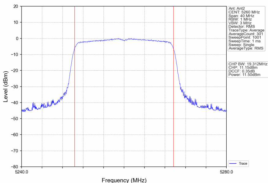
802.11ax(HEW20)_LCH_5260MHz_RU242_Left_Ant2_NTNV
