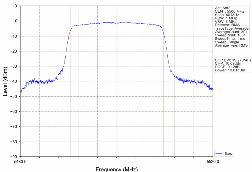
802.11ax(HEW20)_LCH_5500MHz_RU242_Left_Ant2_NTNV
