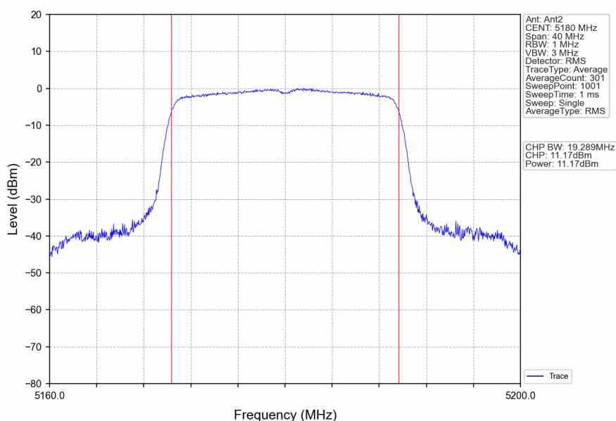
802.11ax(HEW20)_LCH_5180MHz_RU242_Left_Ant2_NTNV
