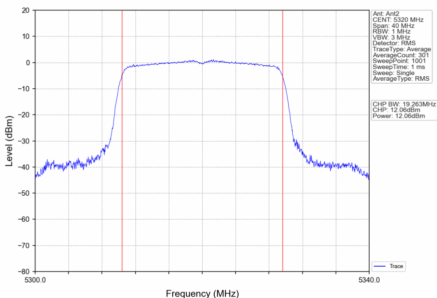
802.11ax(HEW20)_HCH_5320MHz_RU242_Left_Ant2_NTNV
