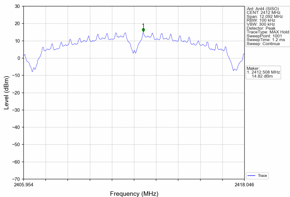
802.11b_LCH_2412MHz_Ant4 (SISO)_NTNV
