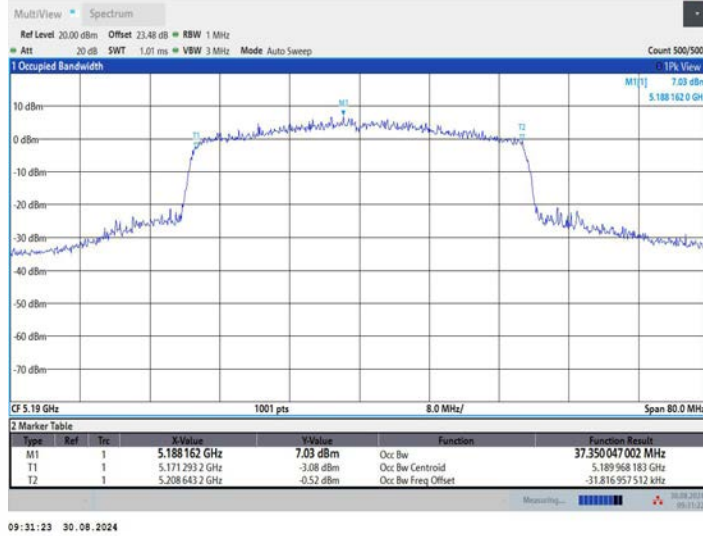
11BE40MIMO_Ant3_5190
