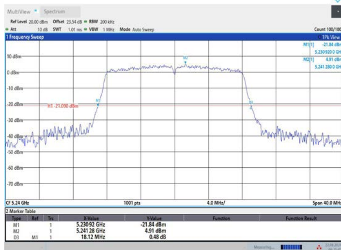
11A_Ant3_5240
