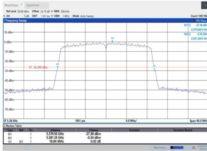
11N20MIMO_Ant3_5580
