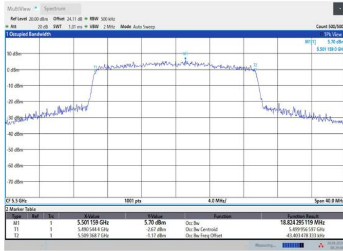
11BE20MIMO_Ant3_5500
