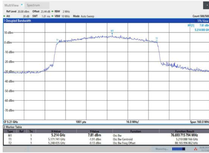
11BE80MIMO_Ant2_5210
