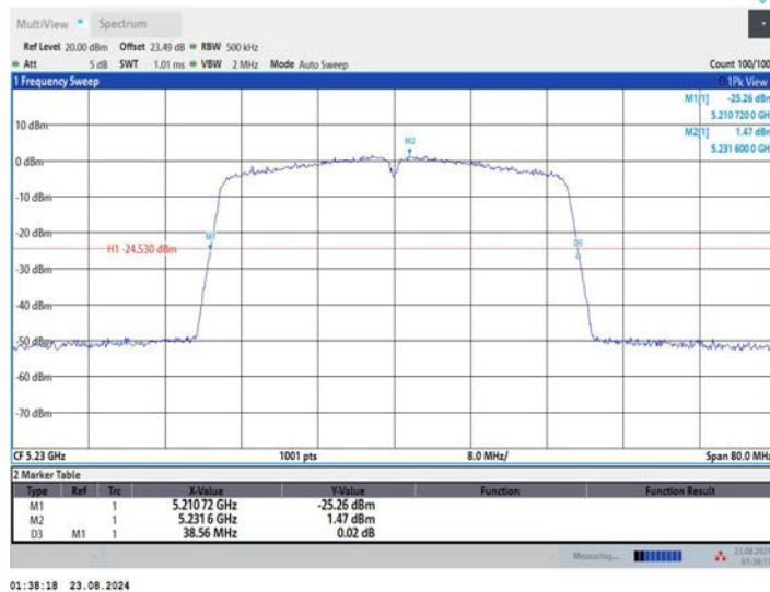
11N40MIMO_Ant2_5230
