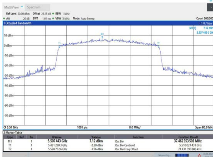
11BE40MIMO_Ant2_5510
