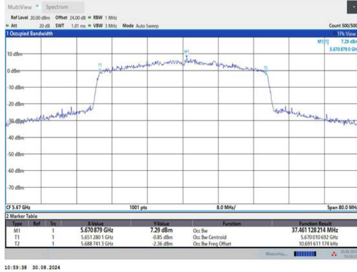
11BE40MIMO_Ant3_5670
