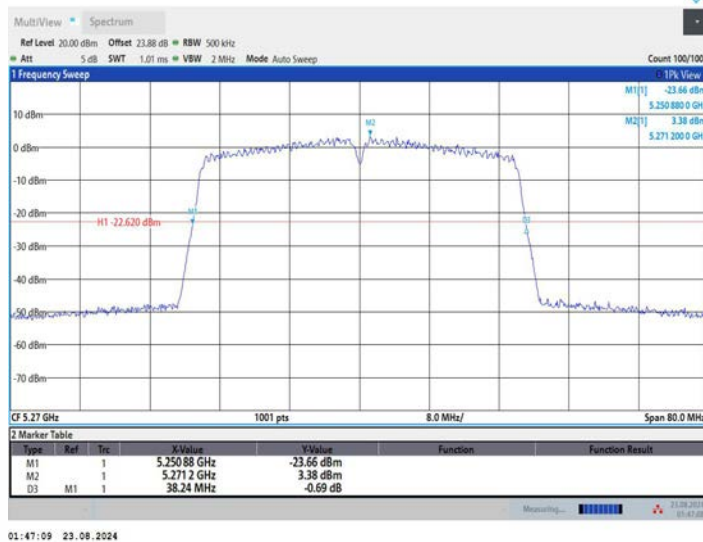
11N40MIMO_Ant3_5270
