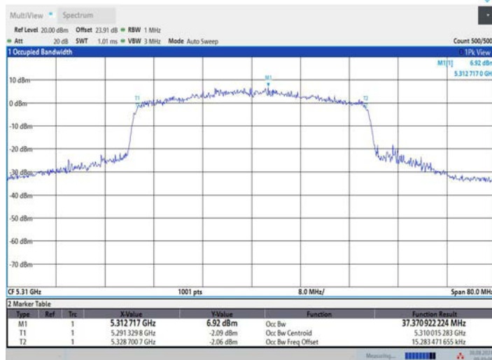
11BE40MIMO_Ant3_5310
