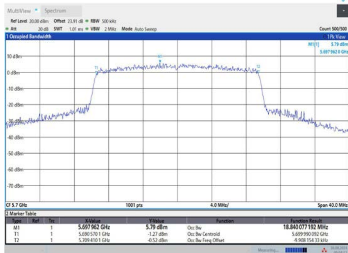
11BE20MIMO_Ant2_5700
