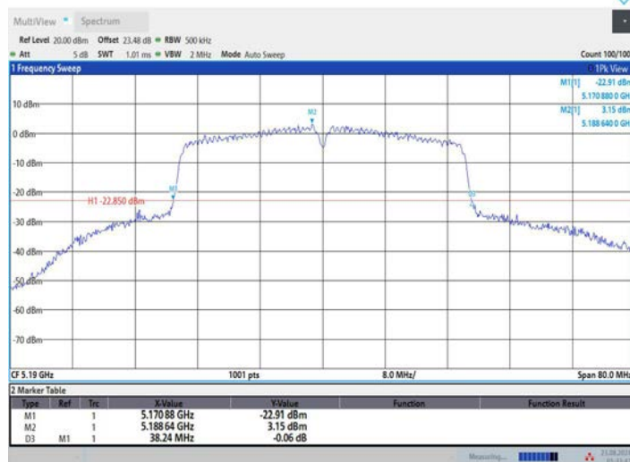
11N40MIMO_Ant3_5190
