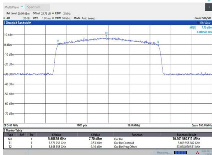
11BE80MIMO_Ant2_5610
