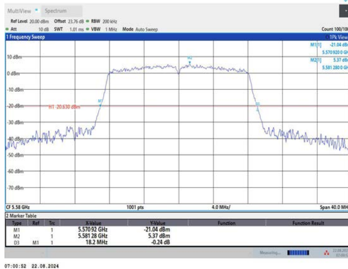
11A_Ant2_5580
