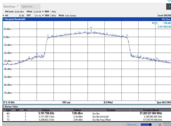
11BE40MIMO_Ant2_5190
