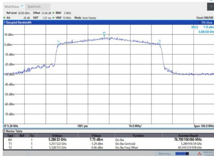
11BE80MIMO_Ant2_5290
