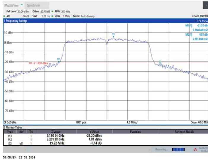
11A_Ant3_5200
