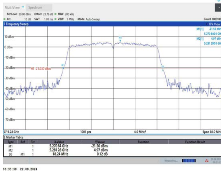
11A_Ant3_5280
