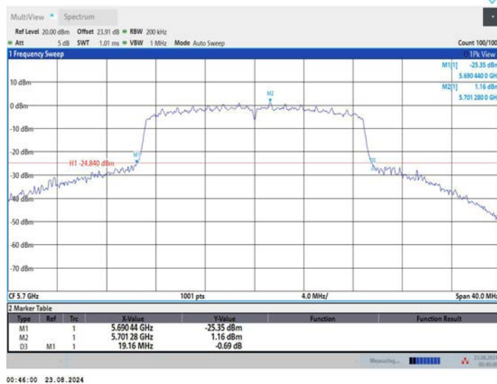
11N20MIMO_Ant3_5700
