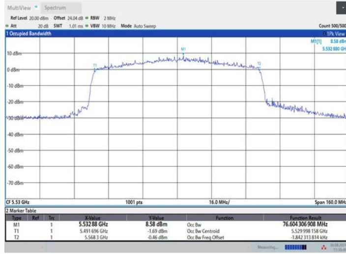
11BE80MIMO_Ant2_5530
