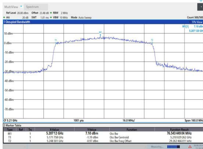
11BE80MIMO_Ant3_5210
