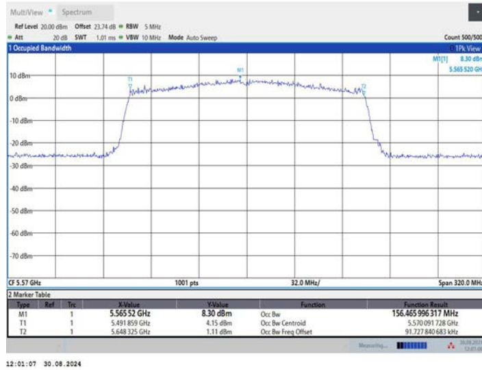
11BE160MIMO_Ant2_5570
