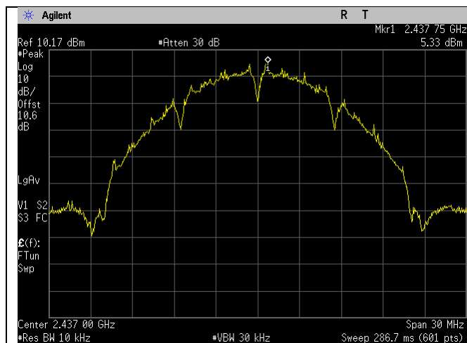
2437MHz_b-mode
