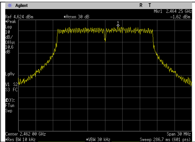
2462MHz_g-mode
