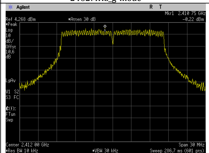
2412MHz_g-mode
