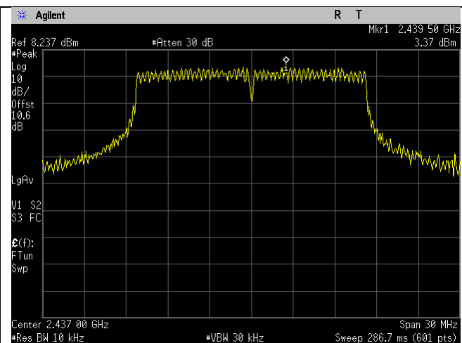
2437MHz_g-mode
