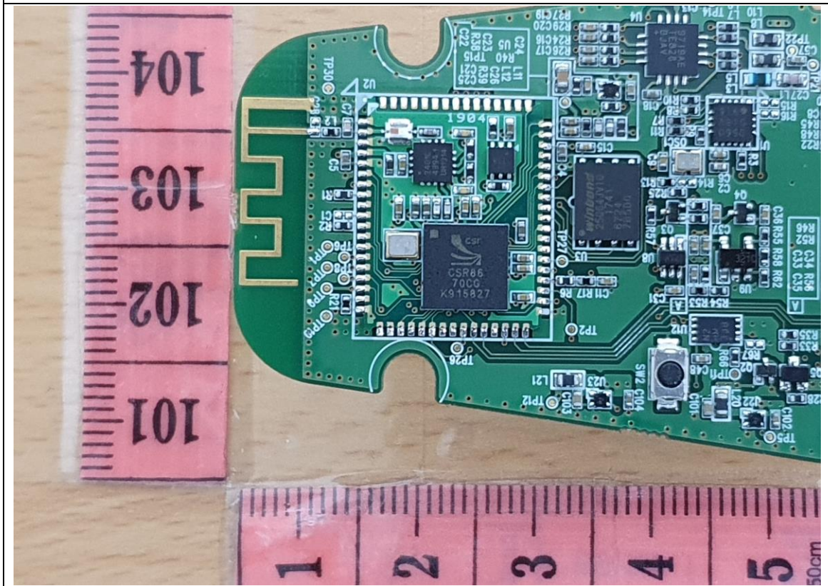
Bluetooth Module & Antenna
