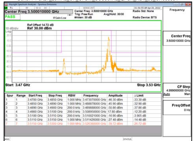
Band77-Part27_20MHz_CP_OFDM_SCS30kHz_OPSK_RB1_50_CH633334
