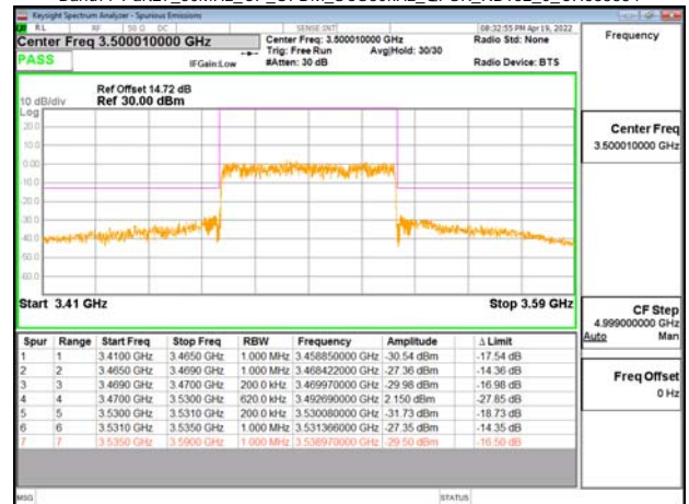
Band77-Part27_60MHz_CP_OFDM_SCS30kHz_QPSK_RB162_0_CH633334
