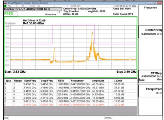
Band77-Part27_20MHz_DFT_s_OFDM_SCS30kHz_BPSK_RB1_50_CH633334
