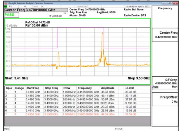
Band77-Part27_40MHz_DFT_s_OFDM_SCS30kHz_BPSK_RB1_105_CH633334
