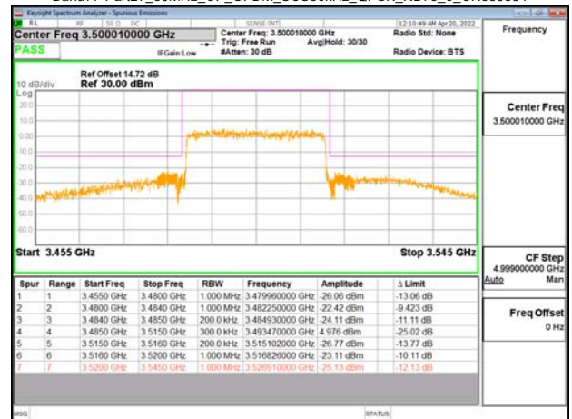
Band77-Part27_30MHz_CP_OFDM_SCS30kHz_QPSK_RB78_0_CH633334
