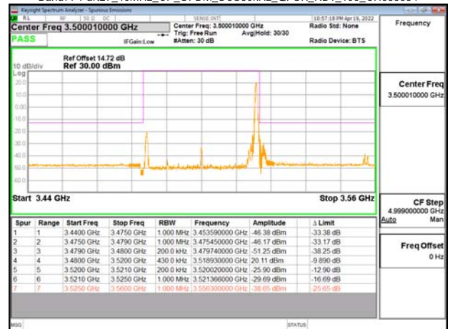
Band77-Part27_40MHz_CP_OFDM_SCS30kHz_QPSK_RB1_105_CH633334
