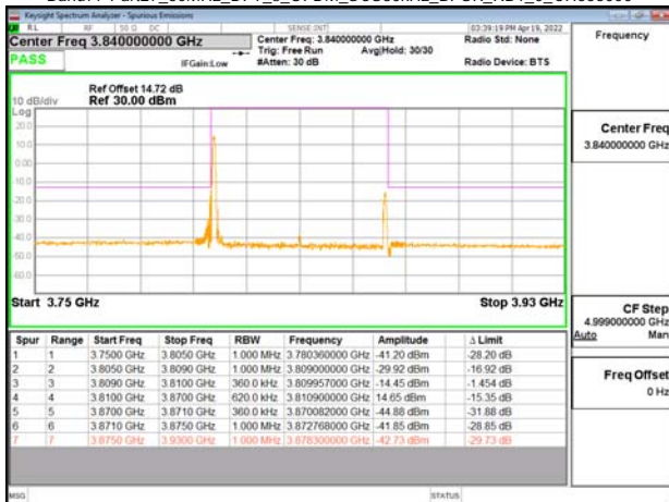
Band77-Part27_60MHz_DFT_s_OFDM_SCS30kHz_BPSK_RB1_0_CH656000
