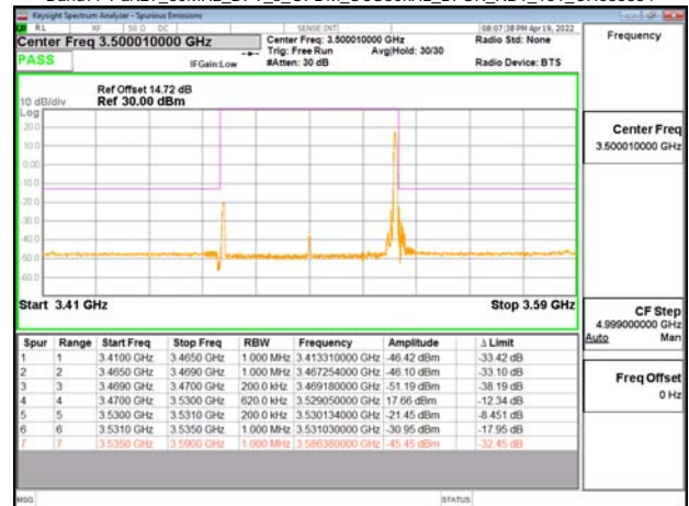
Band77-Part27_60MHz_DFT_s_OFDM_SCS30kHz_BPSK_RB1_161_CH633334
