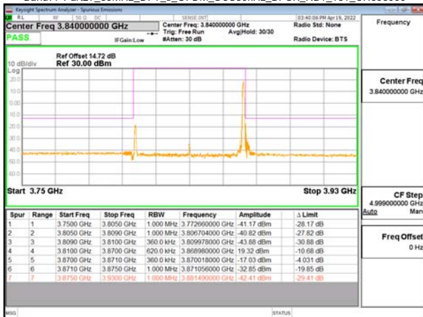
Band77-Part27_60MHz_DFT_s_OFDM_SCS30kHz_BPSK_RB1_161_CH656000
