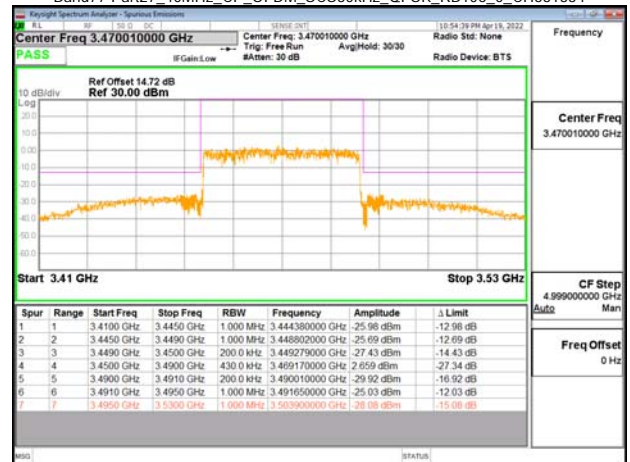
Band77-Part27_40MHz_CP_OFDM_SCS30kHz_QPSK_RB106_0_CH633334
