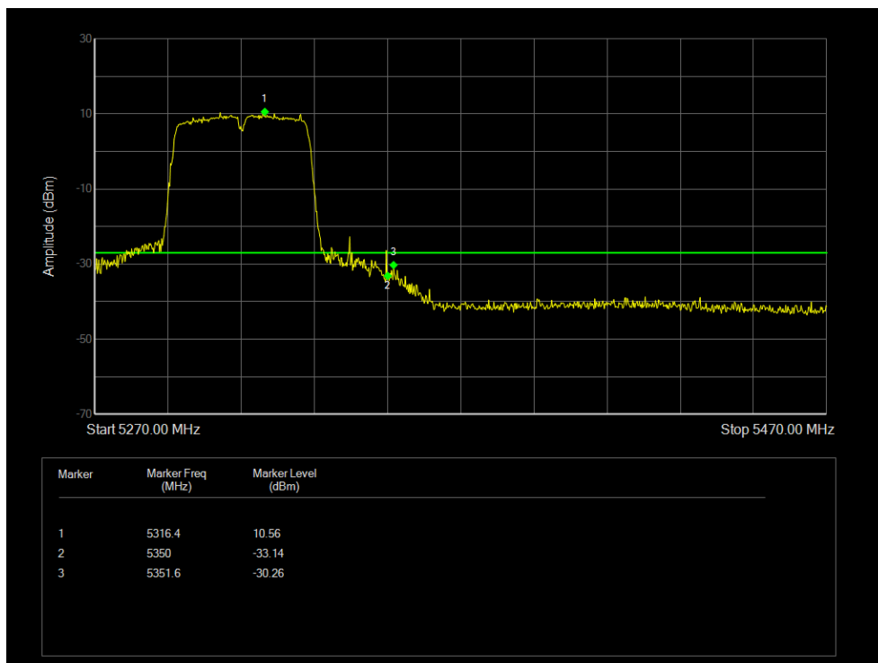
Band Edge NVNT 802.11ax40 5270MHz Low Ant 2
