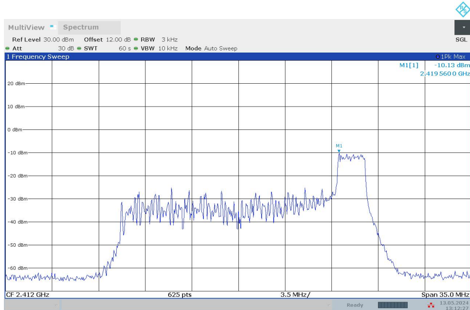
11BE20MIMO_Ant0_2412_52Tone_RU37
