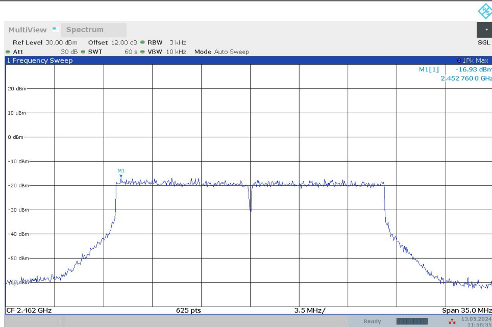
11AX20MIMO_Ant1_2462
