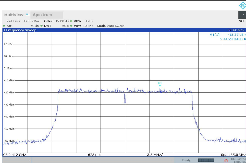
11AX20MIMO_Ant1_2412
