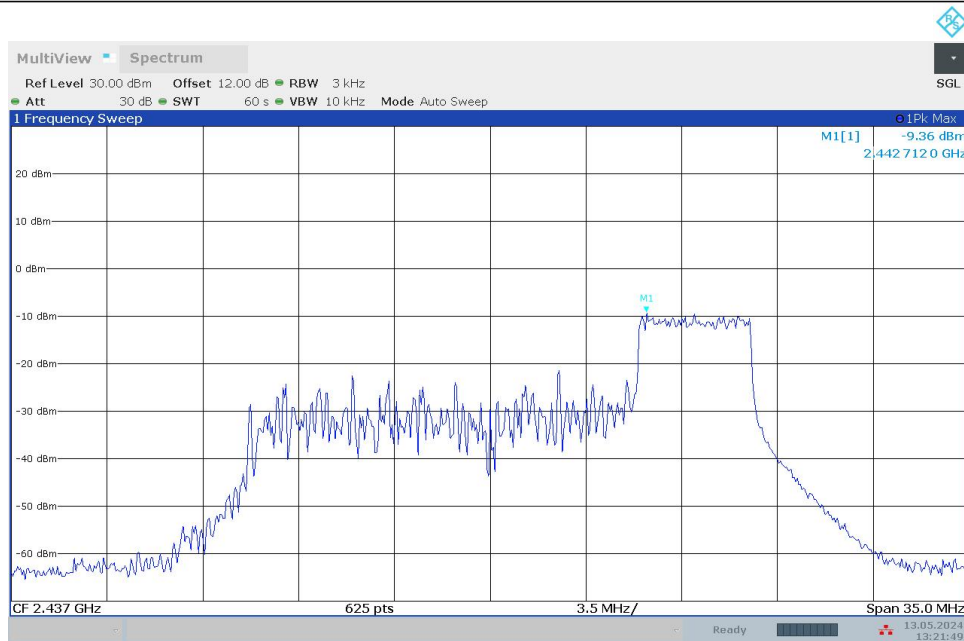
11BE20MIMO_Ant0_2437_106Tone_RU53
