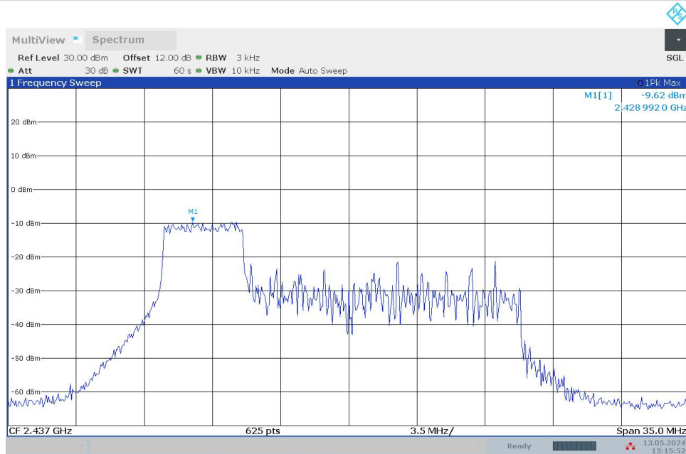
11BE20MIMO_Ant0_2437_52Tone_RU40
