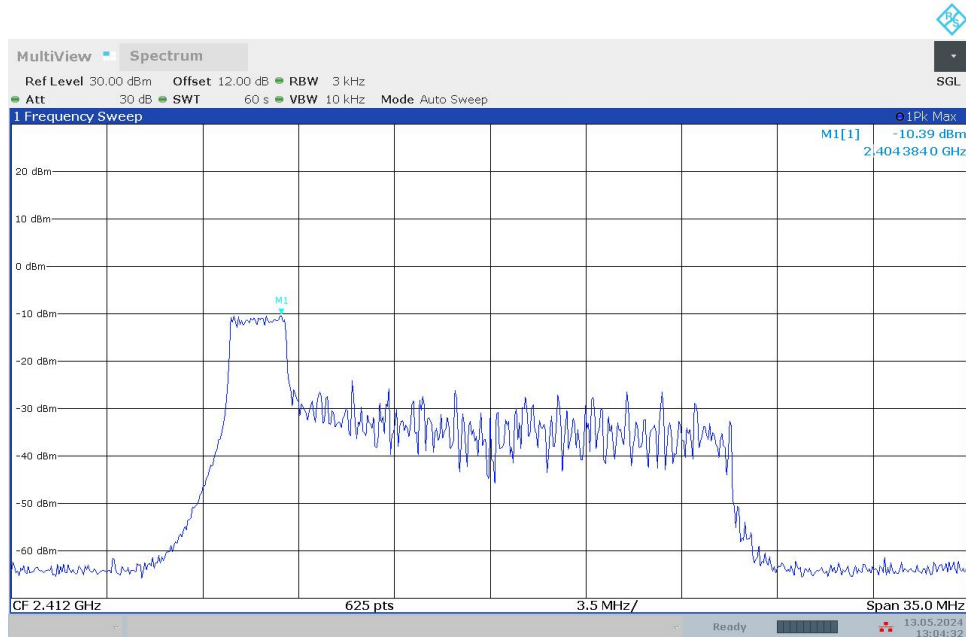
11BE20MIMO_Ant0_2412_26Tone_RU8
