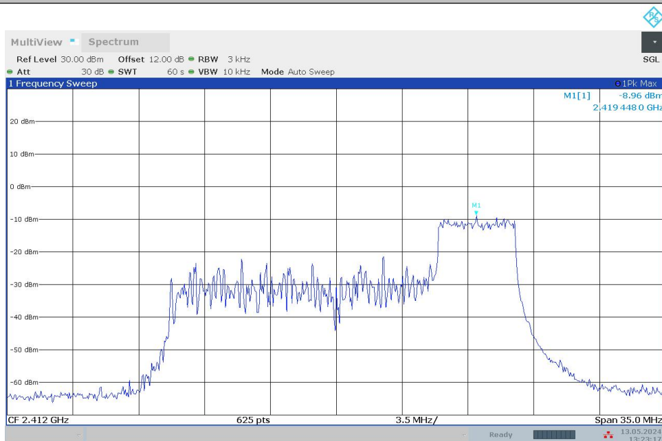
11BE20MIMO_Ant0_2412_52Tone_RU40
