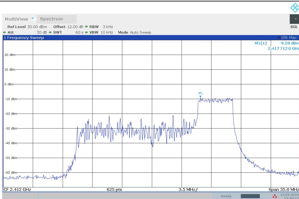
11BE20MIMO_Ant1_2412_52Tone_RU40
