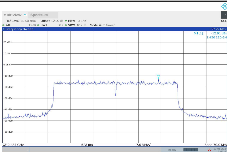
11AX40MIMO_Ant0_2437
