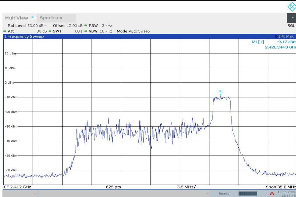
11BE20MIMO_Ant1_2412_52Tone_RU37
