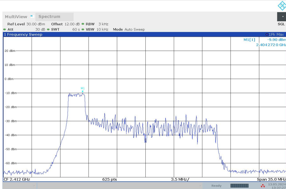
11BE20MIMO_Ant1_2412_26Tone_RU8
