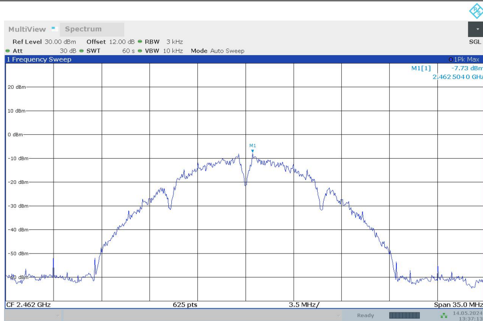
11B- MIMO_Ant0_2462
