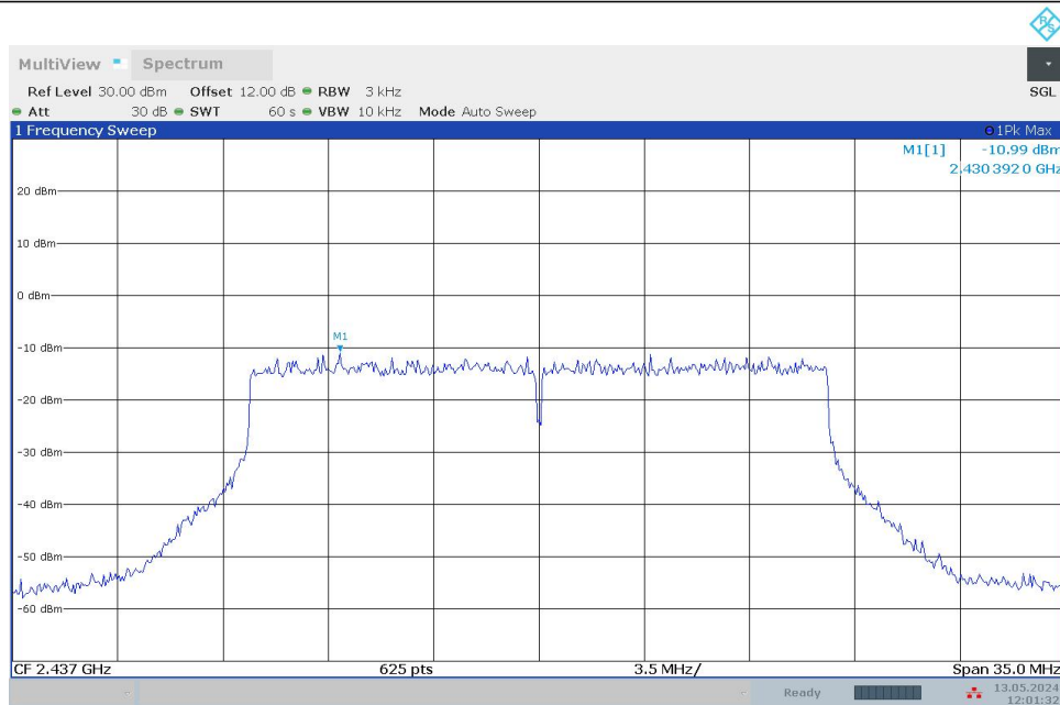
11AX20MIMO_Ant1_2437
