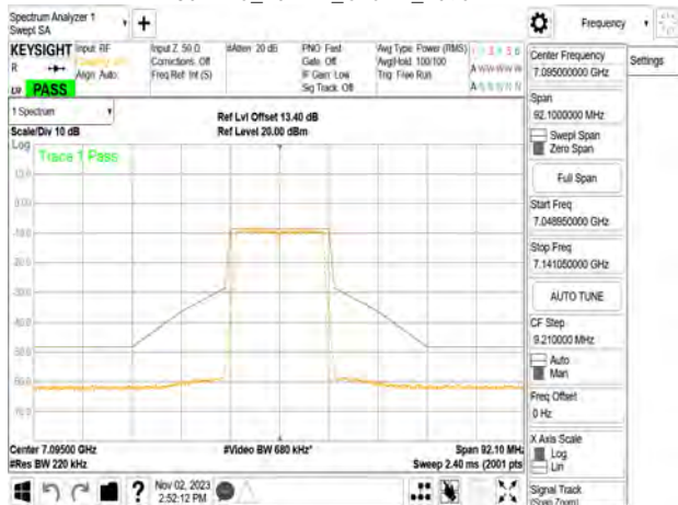
802.11a_20MHz_Chain2_7095MHz
