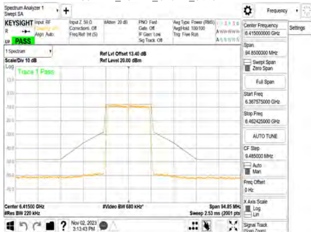
802.11n_20MHz_Chain2_6415MHz
