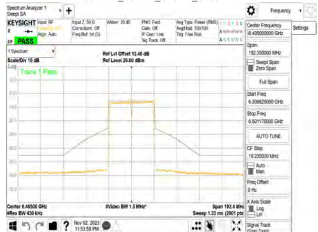
802.11n_40MHz_Chain1_6405MHz
