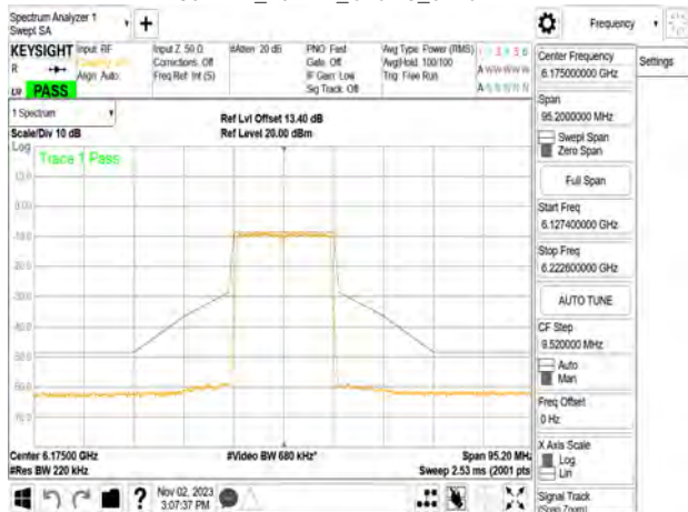
802.11n_20MHz_Chain3_6175MHz
