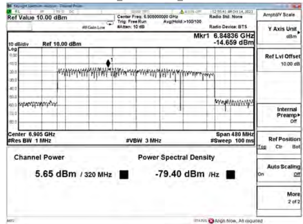
Channel Power+PSD_802.11be320_802.11be320 6905MHz
