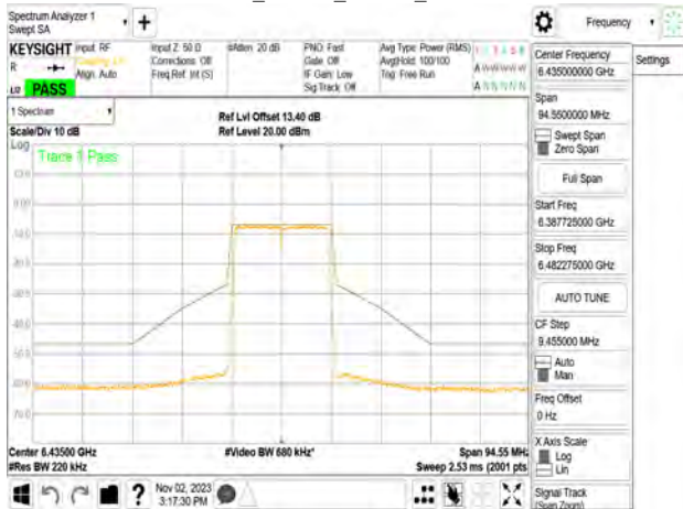
802.11n_20MHz_Chain1_6435MHz
