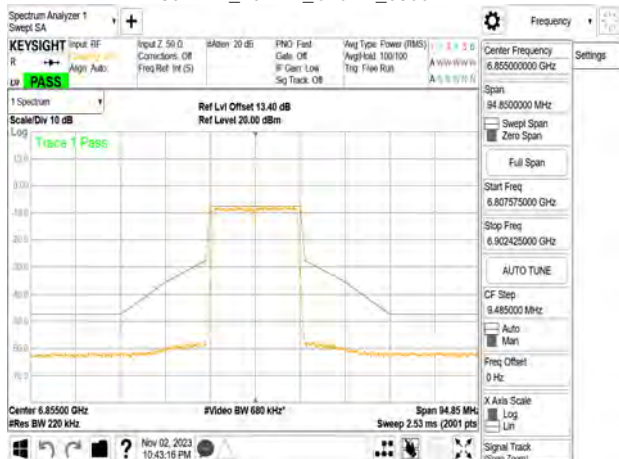
802.11n_20MHz_Chain2_6855MHz
