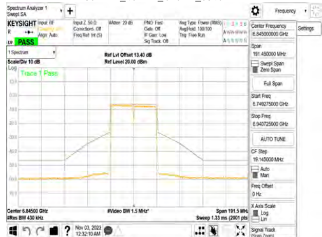
802.11n_40MHz_Chain1_6845MHz
