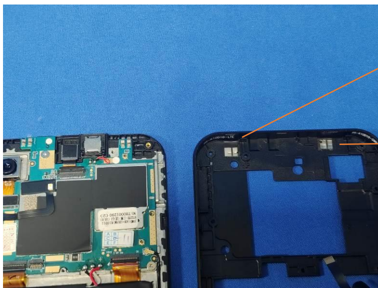
BT/WIFI antenna
