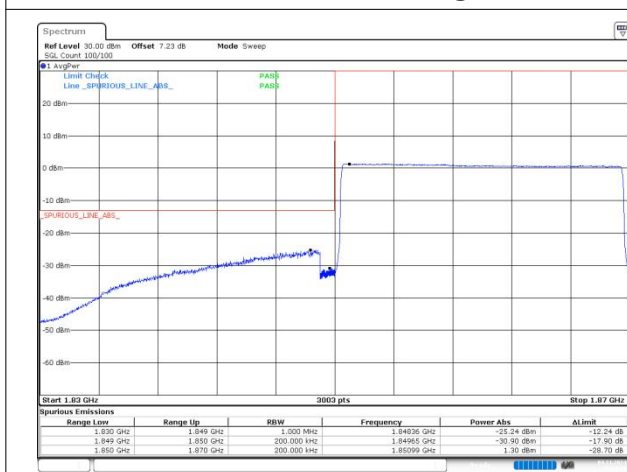
n25 SCS=15kHz DFT_256QAM BW=20MHz LowChannel=372000 RB=1@0
