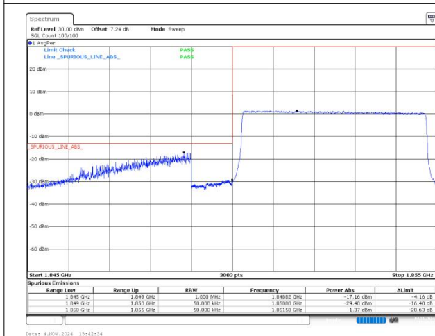
n25 SCS=15kHz CP_QPSK BW=5MHz LowChannel=370500 RB=25@0
