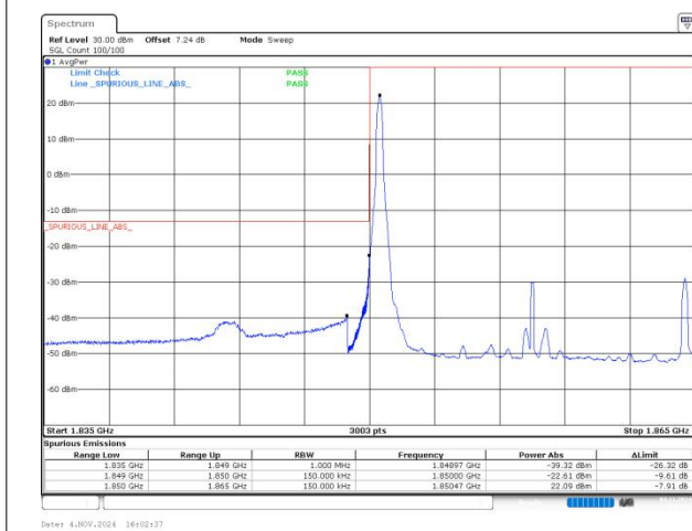
n25 SCS=15kHz DFT_BPSK BW=15MHz LowChannel=371500 RB=1@0
