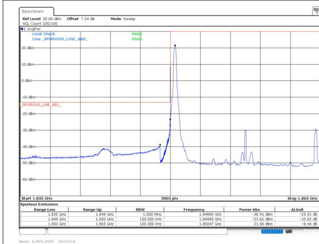
n25 SCS=15kHz DFT_QPSK BW=15MHz LowChannel=371500 RB=1@0
