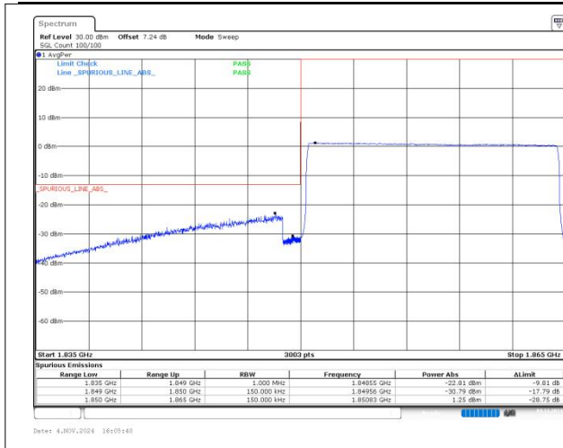
n25 SCS=15kHz CP_QPSK BW=15MHz LowChannel=371500 RB=79@0
