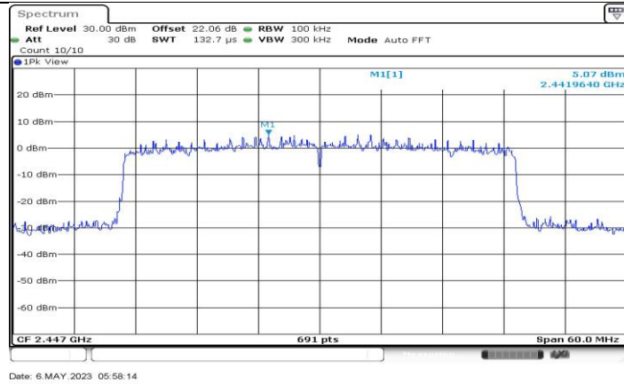
11AX40MIMO_Ant2_2447_0-Reference
