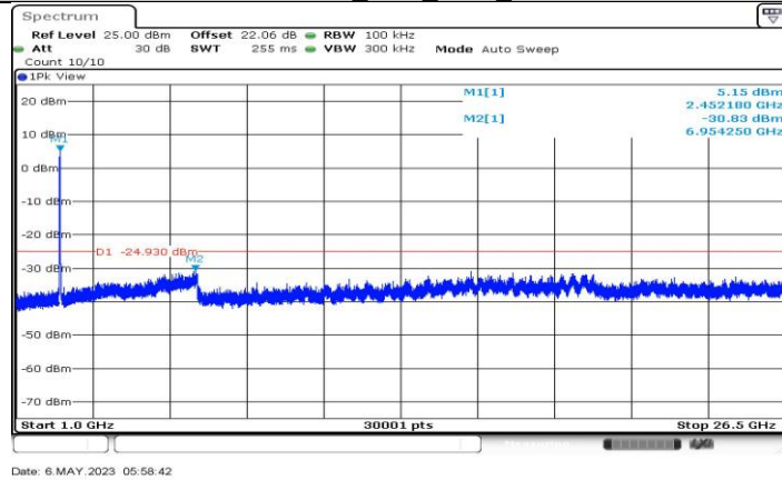
11AX40MIMO_Ant2_2447_1000-26500
