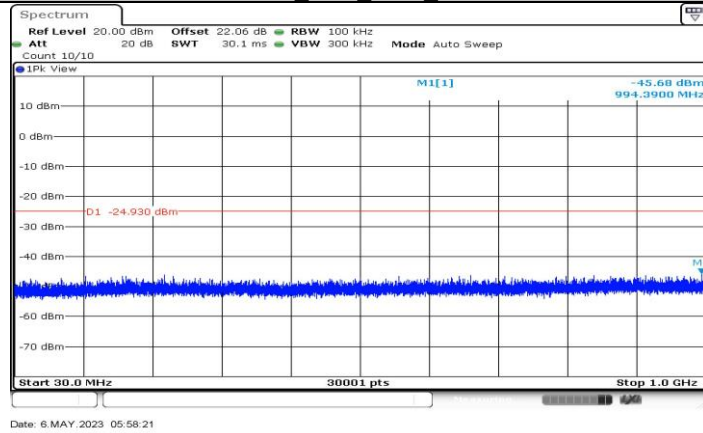
11AX40MIMO_Ant2_2447_30-1000
