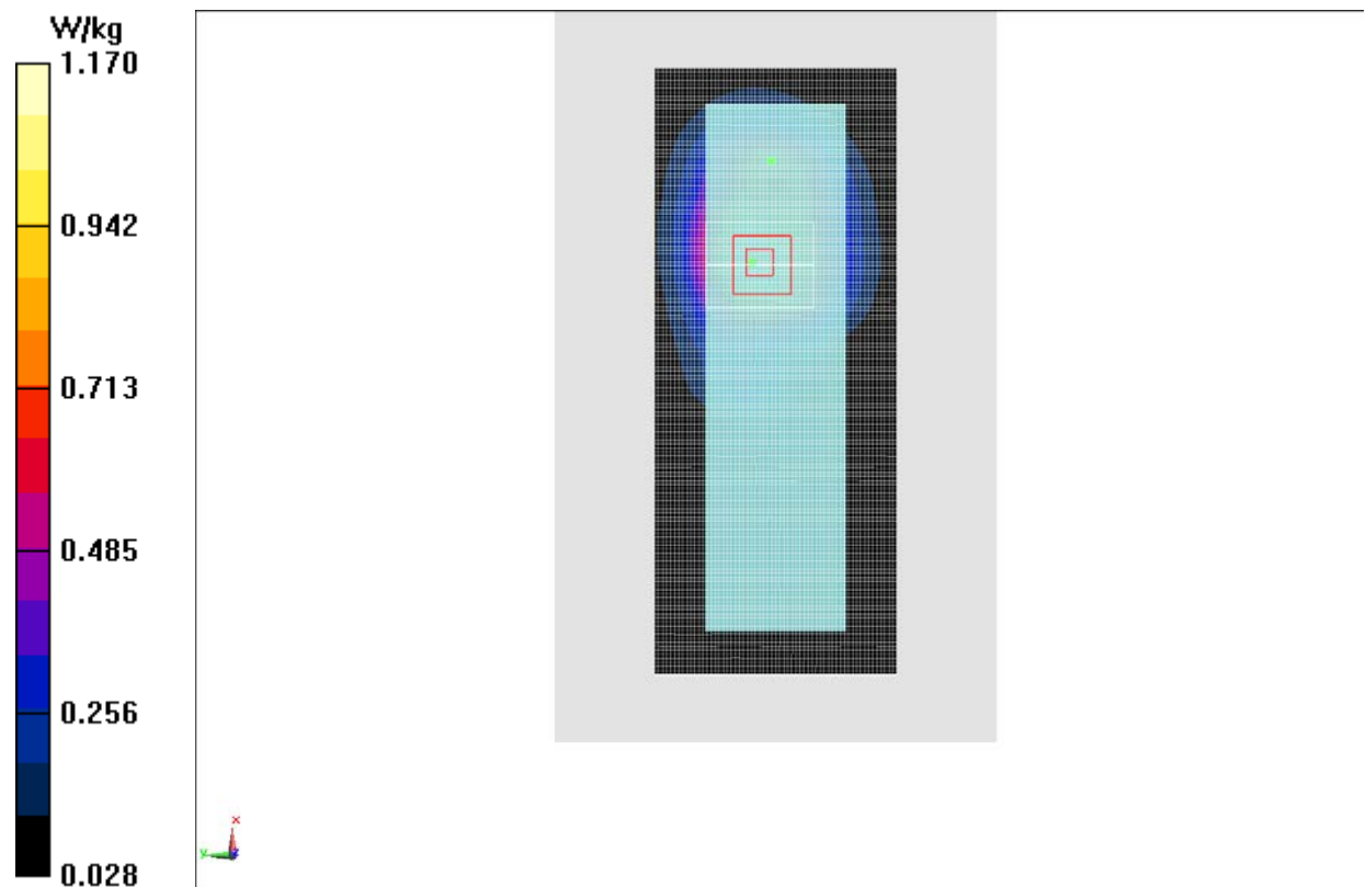
Fig.10 WCDMA1900
