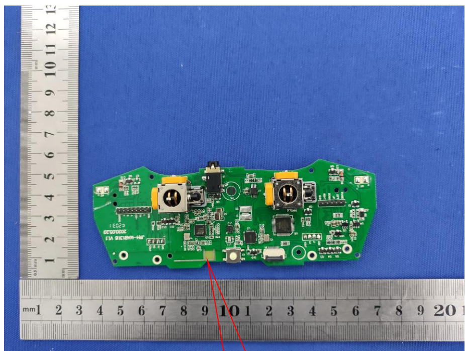
Antenna
