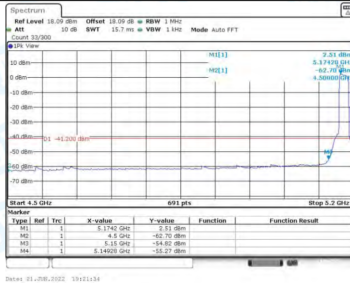
11N20MIMO_Ant2_Low_5180_AV
