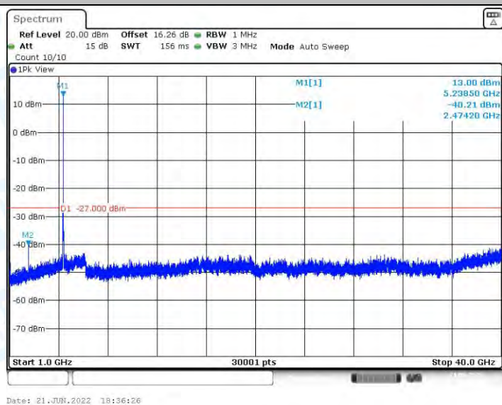
11A_Ant2_5240_1000~40000
