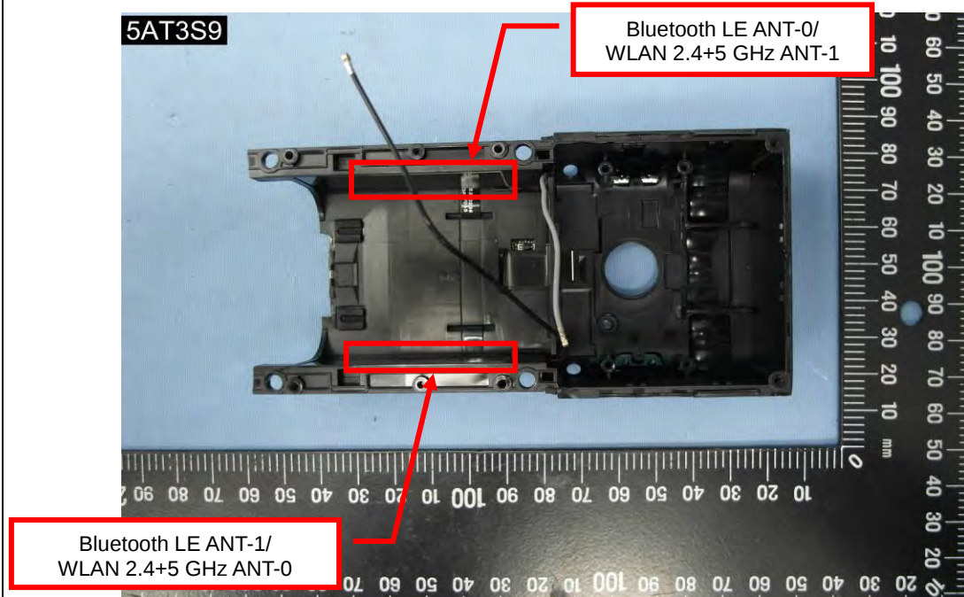
EUT Photo (64)
