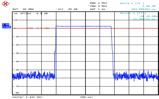
GFSK_Hopping_DH1 0.404ms
