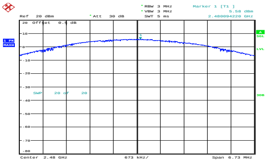
\pi/4 -DQPSK_High 5.58dBm
