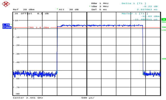
\pi/4 -DQPSK_Hopping_2DH5 2.937ms
