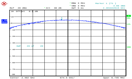
\pi/4 -DQPSK_Low 4.96dBm
