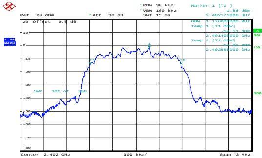
\pi/4 -DQPSK_Low 1.176MHz
