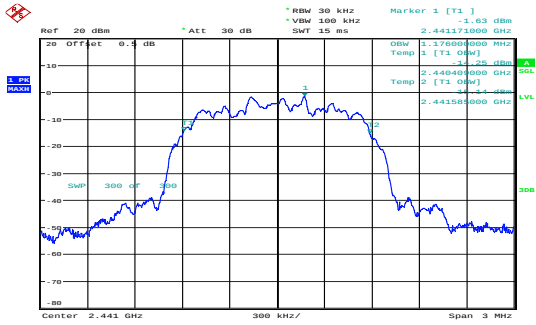
\pi/4 -DQPSK_Middle 1.176MHz
