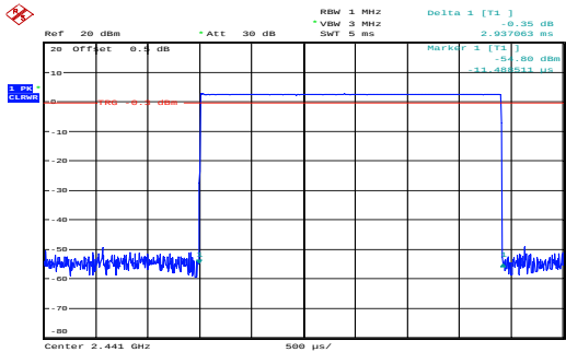
GFSK_Hopping_DH5 2.937ms
