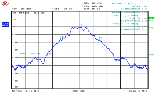
GFSK_High 0.855MHz
