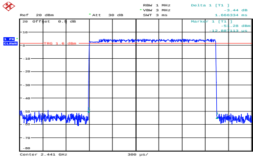
\pi/4 -DQPSK_Hopping_2DH3 1.666ms
