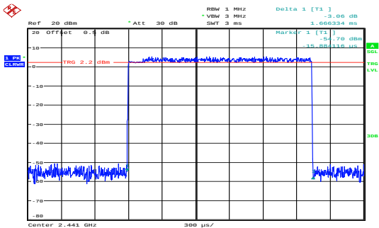
8DPSK_Hopping_3DH3 1.666ms
