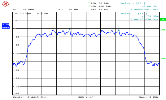
\pi/4 -DQPSK_Middle 1.001MHz
