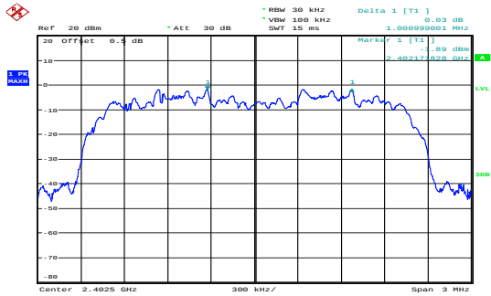
\pi/4 -DQPSK_Low 1.001MHz
