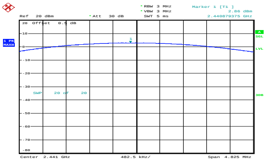
GFSK_Middle 2.86dBm
