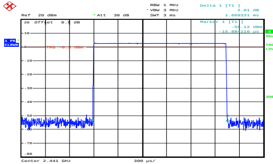
GFSK_Hopping_DH3 1.669ms
