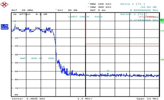
\pi/4 -DQPSK_Hopping_Upper 54.83dB
