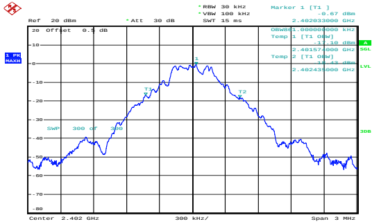
GFSK_Low 0.861MHz
