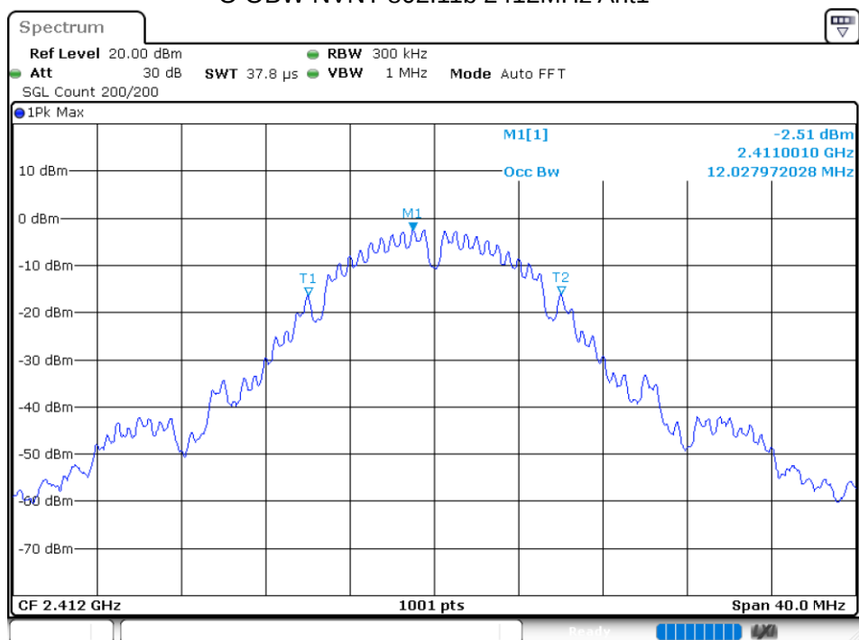
O OBW NVNT 802.11b 2412MHz Ant1
