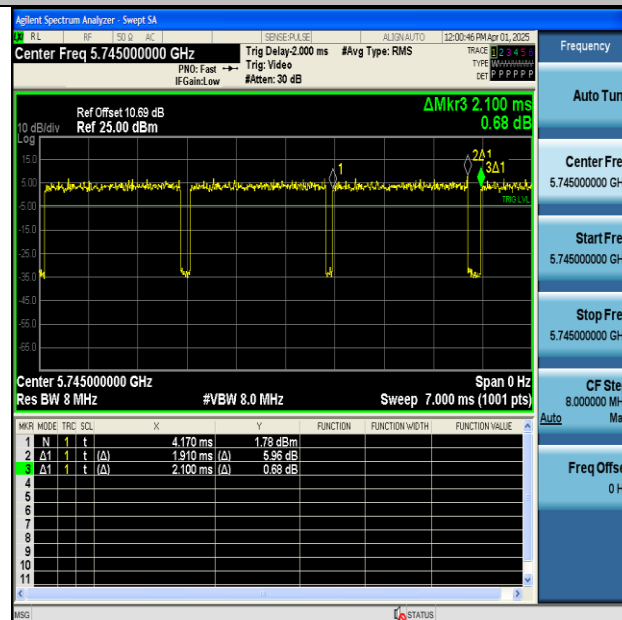
NTNV-11N20MIMO-Ant1-5745
