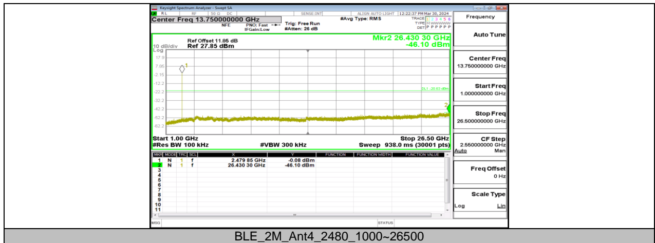
BLE_2M_Ant4_2480_1000~26500
