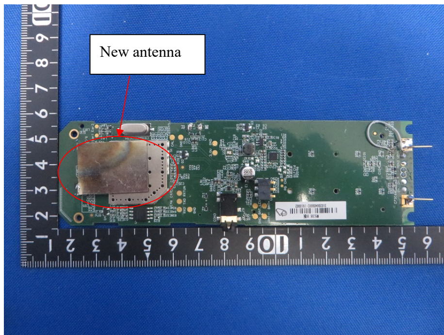
(6) EUT Photo
