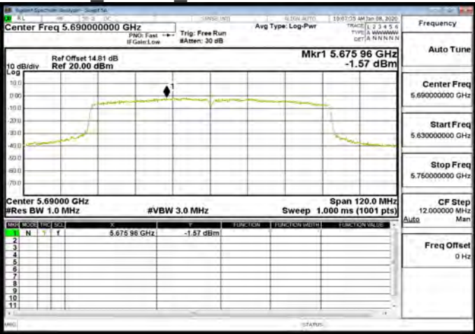
802.11ac 80MHz 5690MHz UNII 2C
