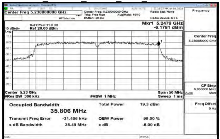
IC 802.11n 40MHz Main 5230MHz
