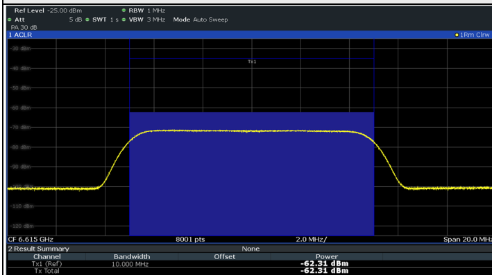
802.11ax (HE20) / CH133
