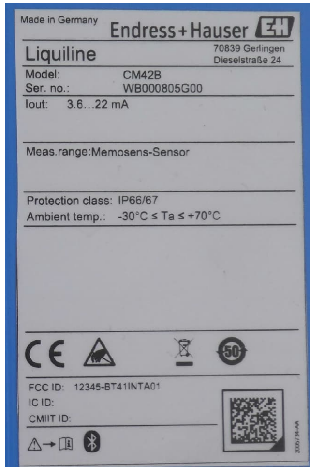
EUT – type plate
