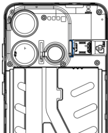
Fente pour la carte SIM
