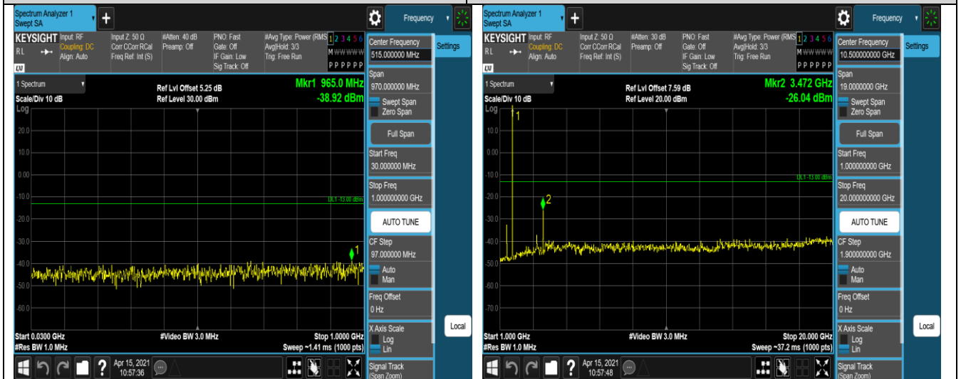
Band4-1.4MHz-QPSK-20393-1RB#0-Range1:30~1000MHz
