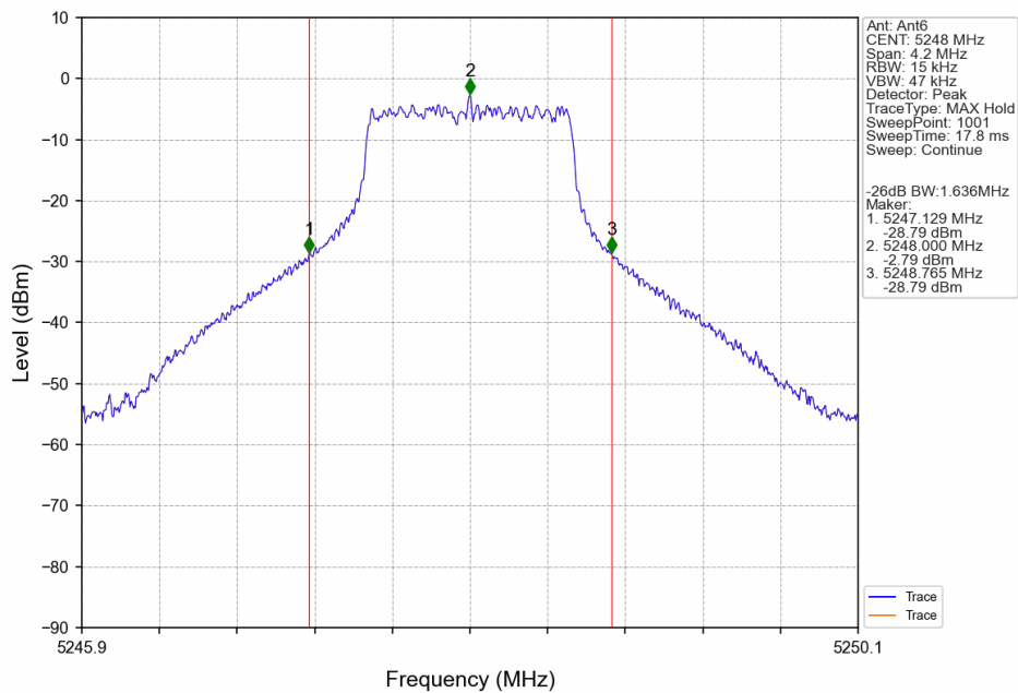
1.4M_HCH_5248MHz_Ant6_NTNV
