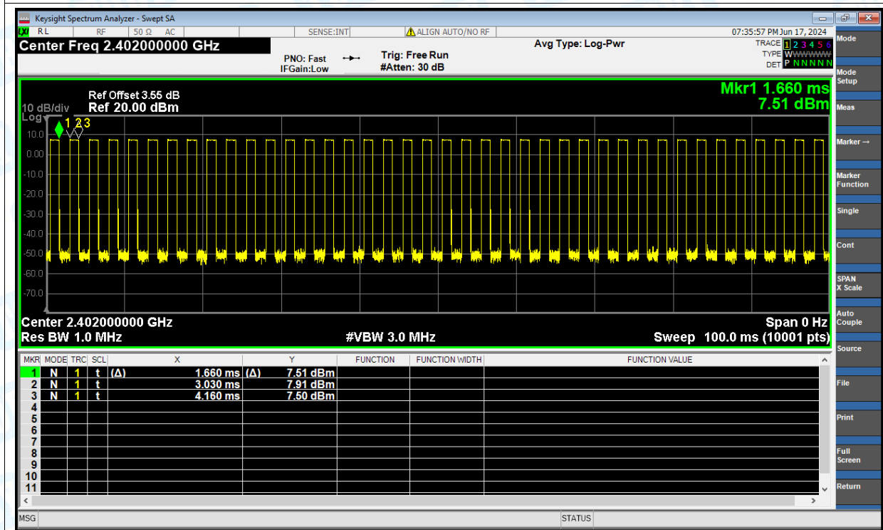
Duty Cycle NVNT BLE 2Mbps 2402MHz Ant1
