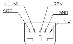
SECTION A (コネクタピン配列) 勘合相手部品:854-9078-50
