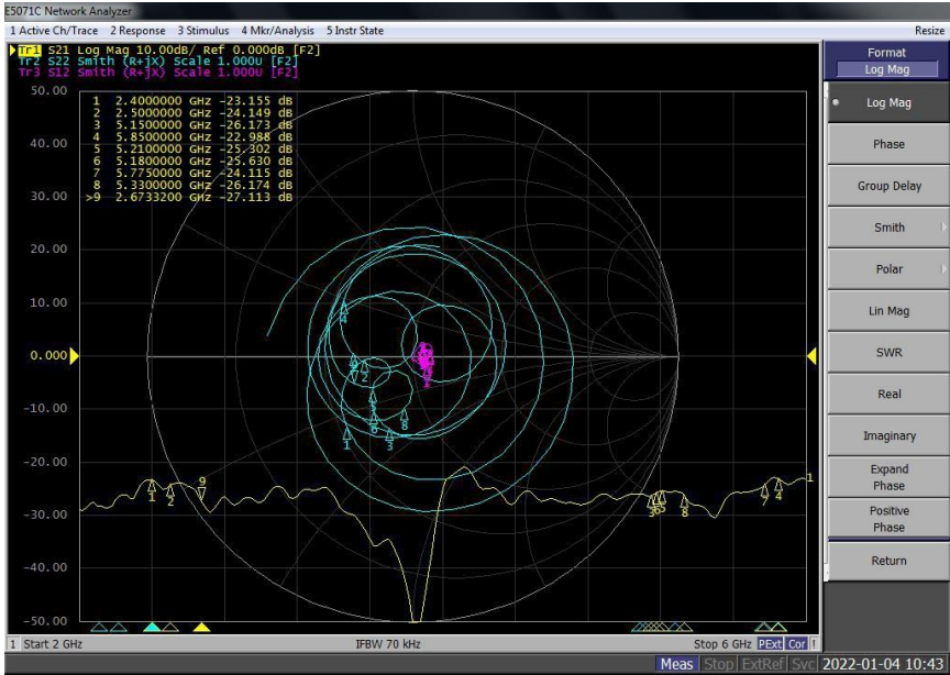
天线隔离度值 (一) Isolation(1)
