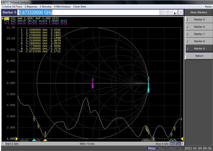
BT 天线驻波比值 VSWR
