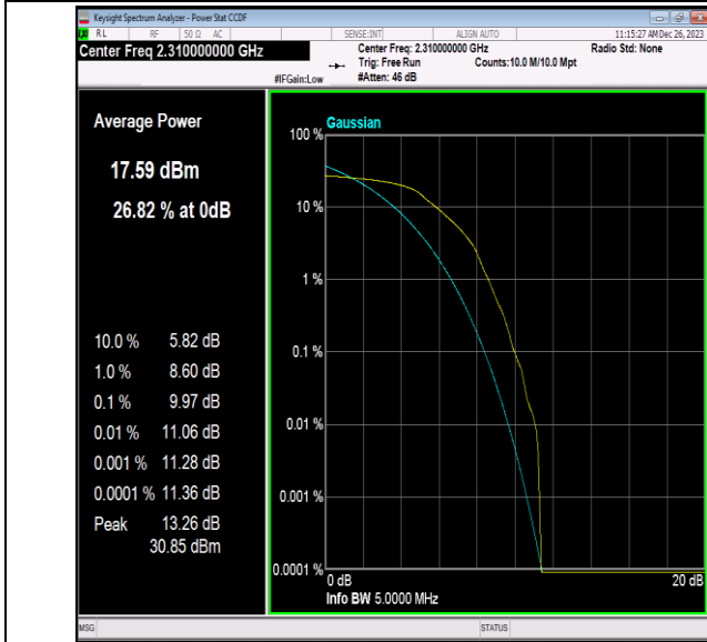
40(2305-2315)-5MHz-QPSK-38750-1RB#0-PASS
