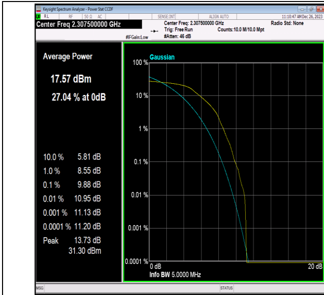
40(2305-2315)-5MHz-QPSK-38725-1RB#0-PASS
