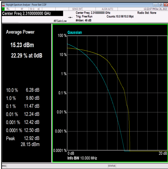
40(2305-2315)-10MHz-64QAM-38750-1RB#0-PASS
