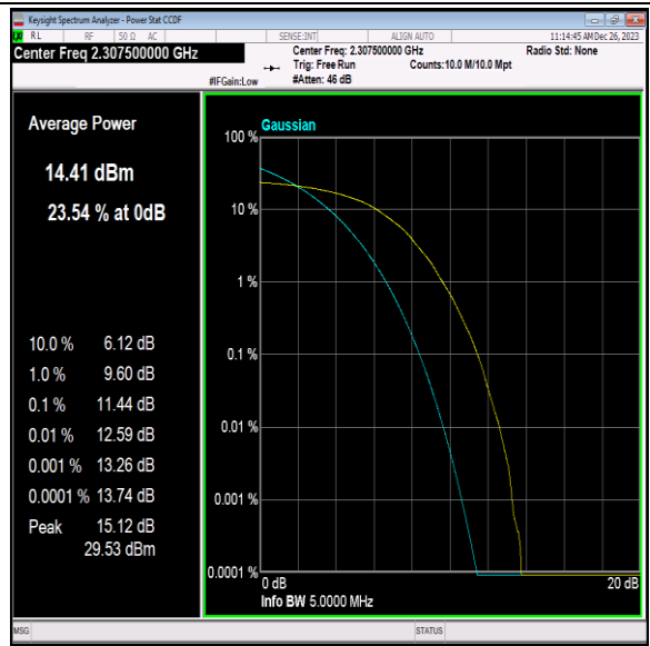
40(2305-2315)-5MHz-64QAM-38725-25RB#0-PASS
