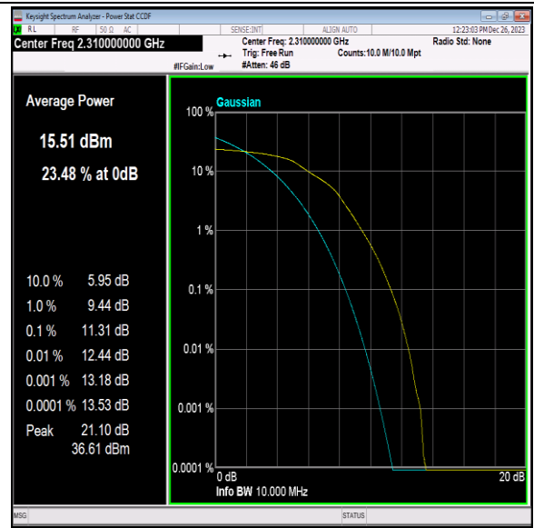
40(2305-2315)-10MHz-16QAM-38750-50RB#0-PASS
