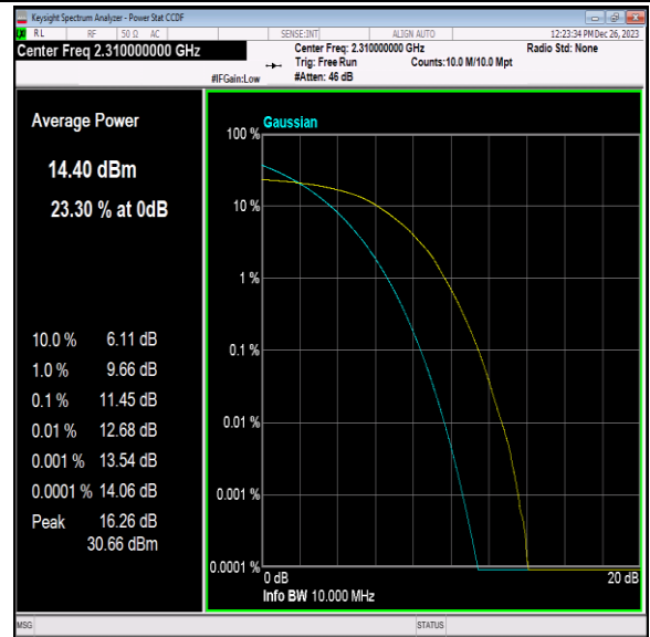
40(2305-2315)-10MHz-64QAM-38750-50RB#0-PASS
