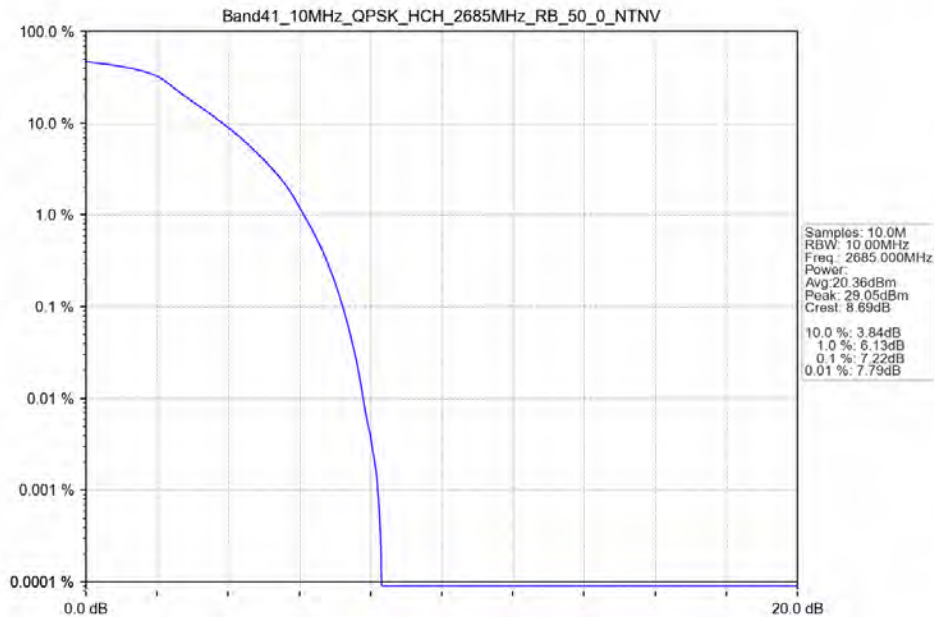
Band41_10MHz_QPSK_HCH_2685MHz_RB_50_0_NTNV
