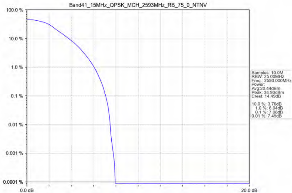
Band41_15MHz_QPSK_MCH_2593MHz_RB_75_0_NTNV
