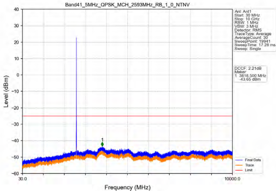
Band41_5MHz_QPSK_MCH_2593MHz_RB_1_0_NTNV
