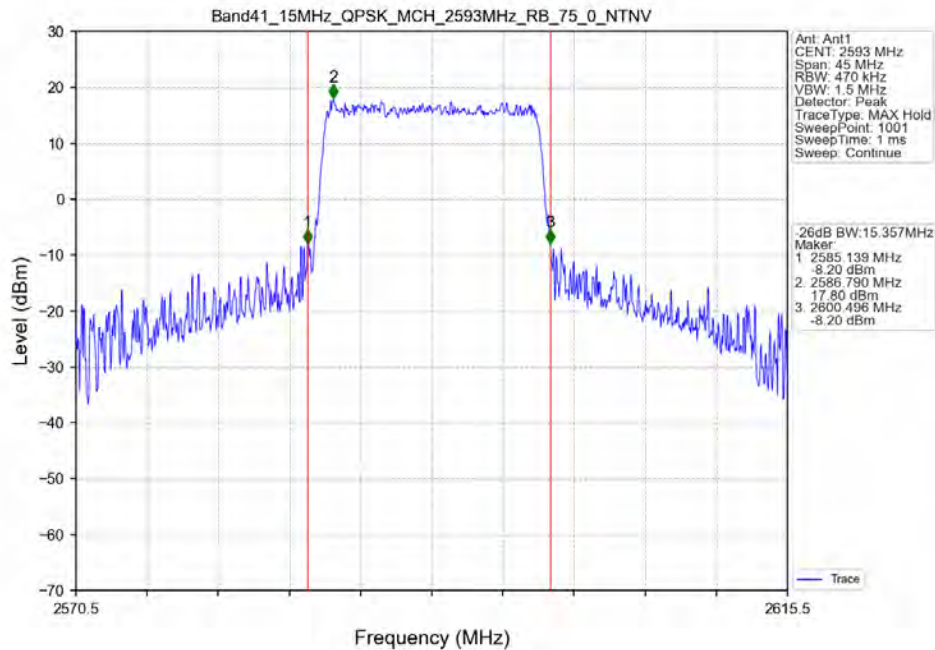
Band41_15MHz_QPSK_MCH_2593MHz_RB_75_0_NTNV
