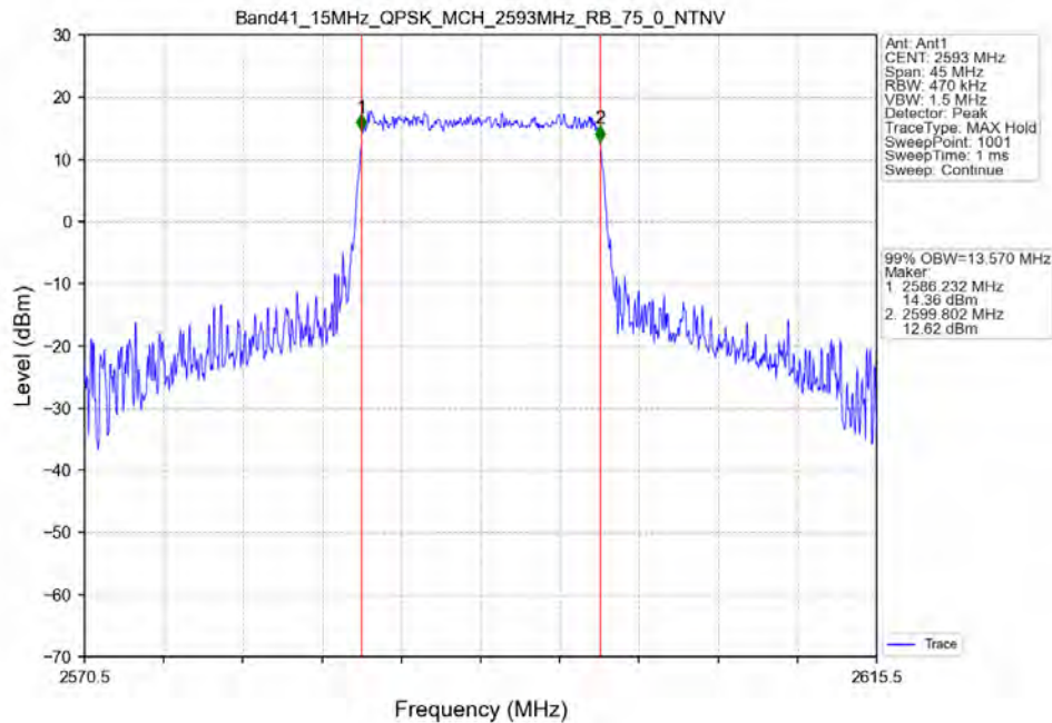
Band41_15MHz_QPSK_MCH_2593MHz_RB_75_0_NTNV
