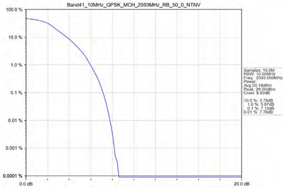
Band41_10MHz_QPSK_MCH_2593MHz_RB_50_0_NTNV
