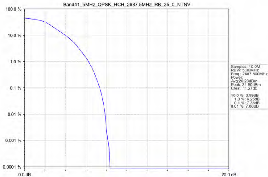
Band41_5MHz_QPSK_HCH_2687.5MHz_RB_25_0_NTNV
