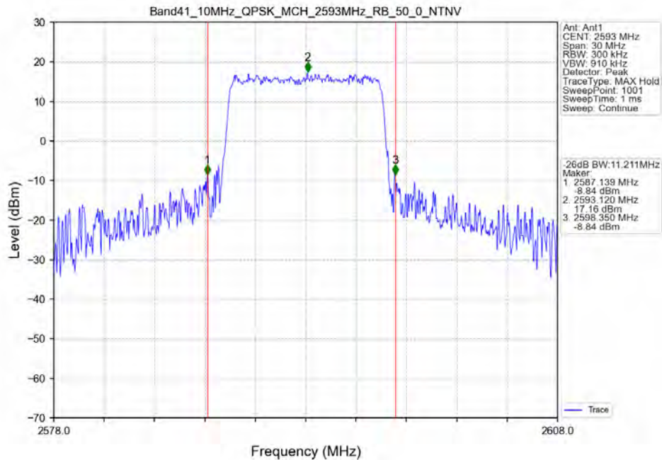
Band41_10MHz_QPSK_MCH_2593MHz_RB_50_0_NTNV
