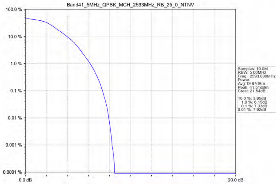
Band41_5MHz_QPSK_MCH_2593MHz_RB_25_0_NTNV
