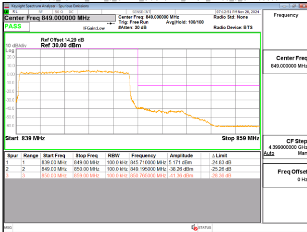
Band5_10MHz_CP_OFDM_SCS15kHz_QPSK_RB1_0_CH168800
