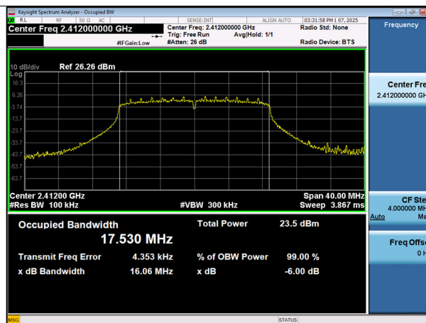
802.11n_HT20-CH 1
