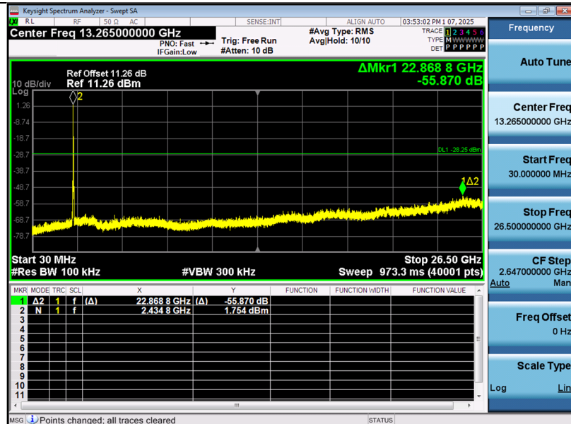
802.11n-CH 6
