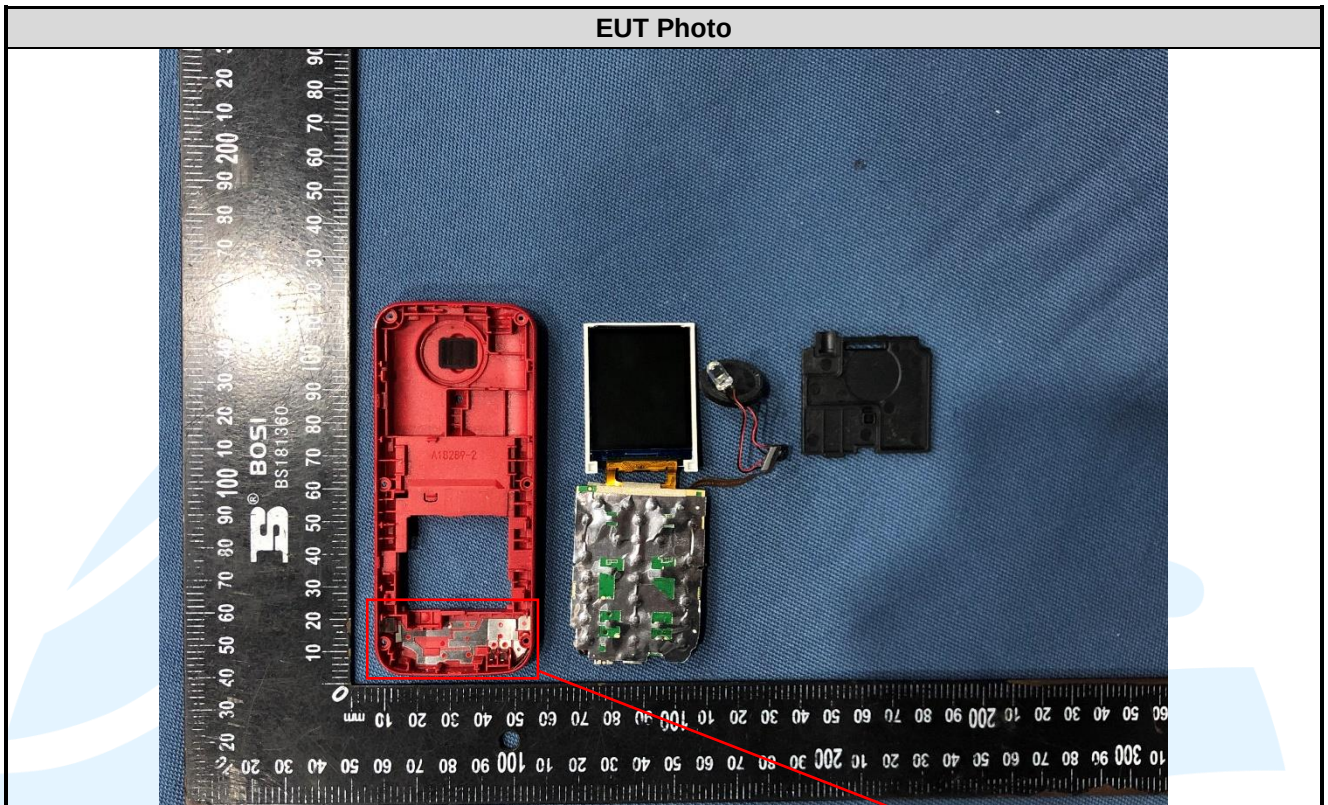
GSM Antenna
